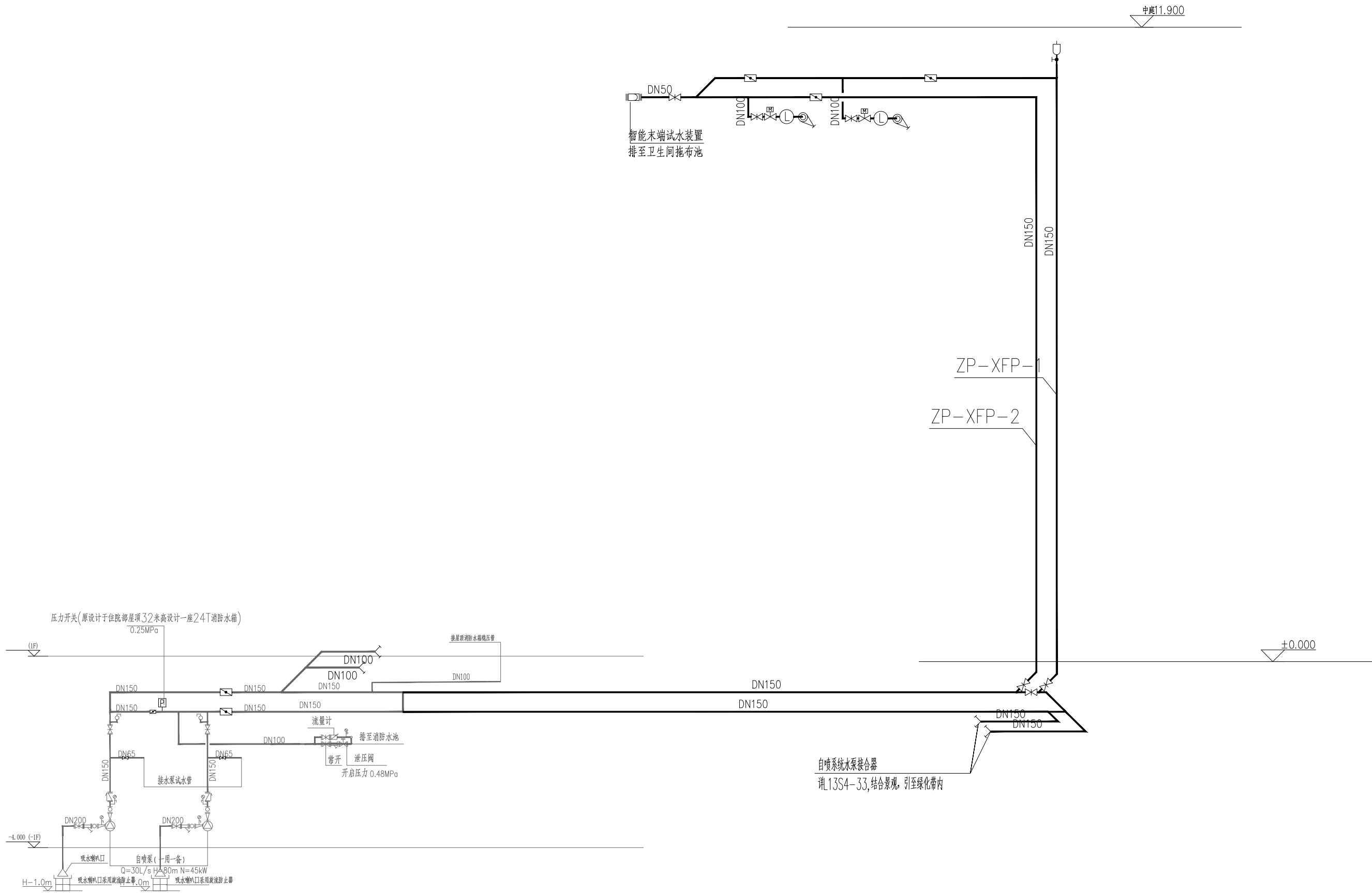
自动喷淋泵系统原理展开图
