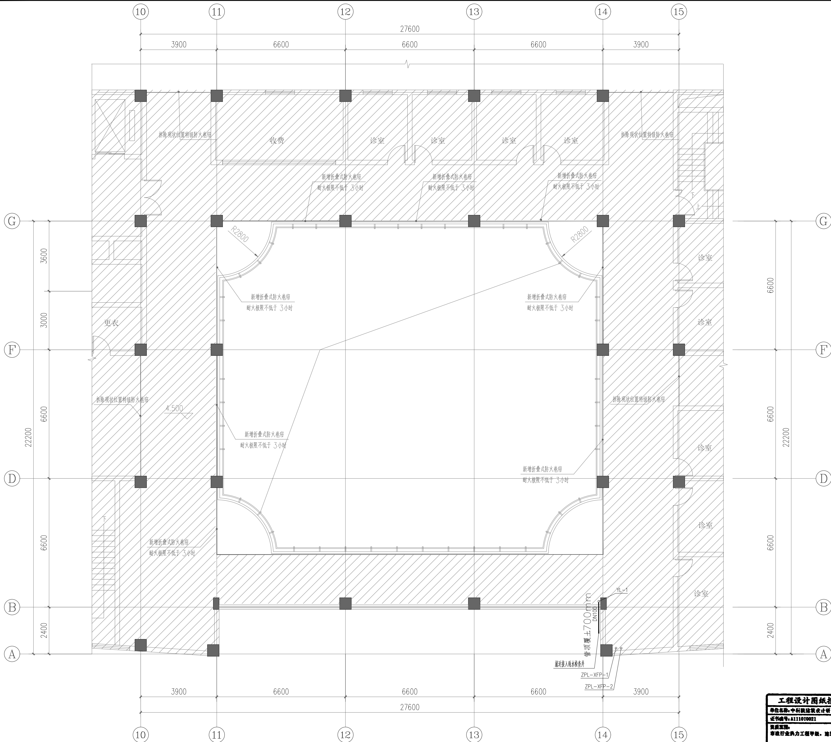
中庭二层给排水、消防平面图 1:100
