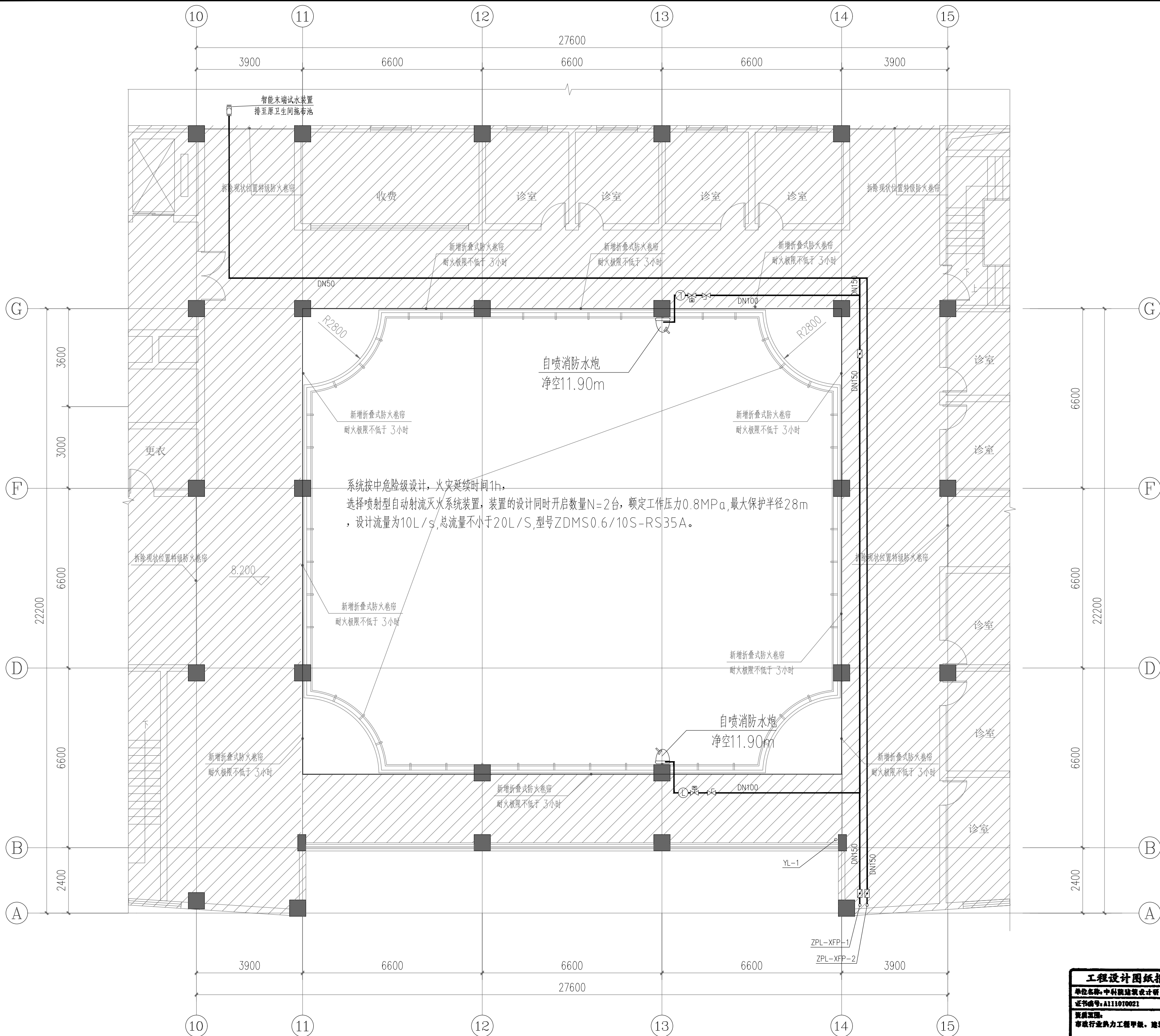
中庭三层给排水、消防平面图 1:100
