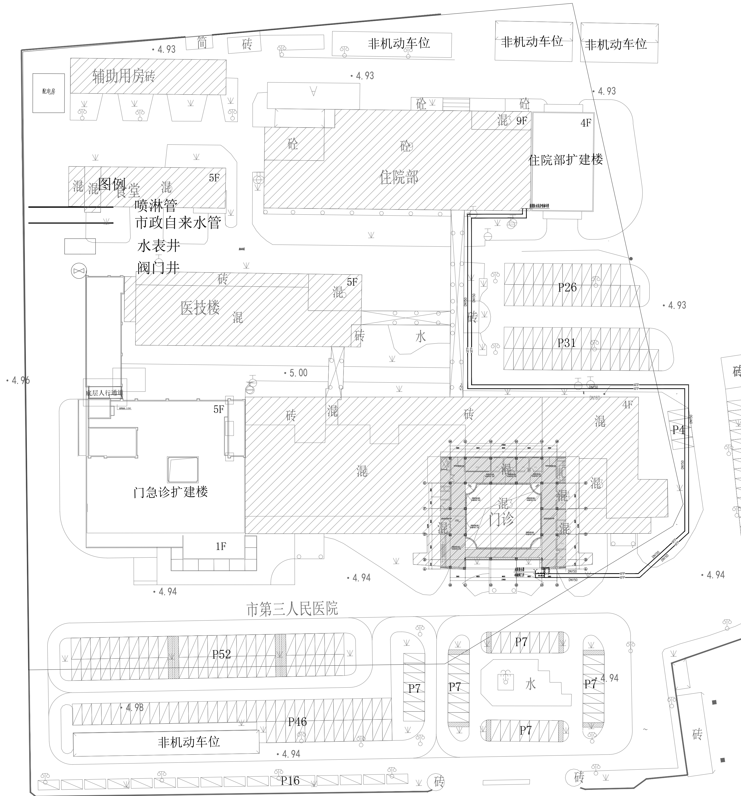
室外给水、消防平面图
