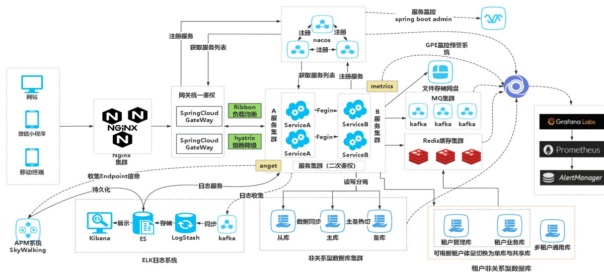
技术架构图
