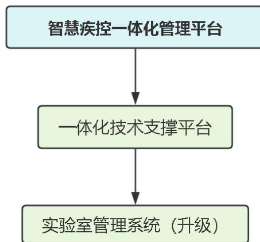
总体架构图
