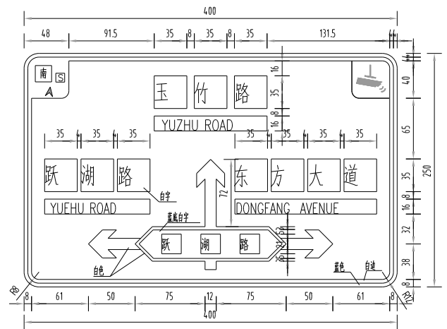
交叉口指路标志牌版面尺寸
