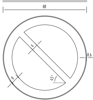
圆形禁令标志牌版面尺寸
