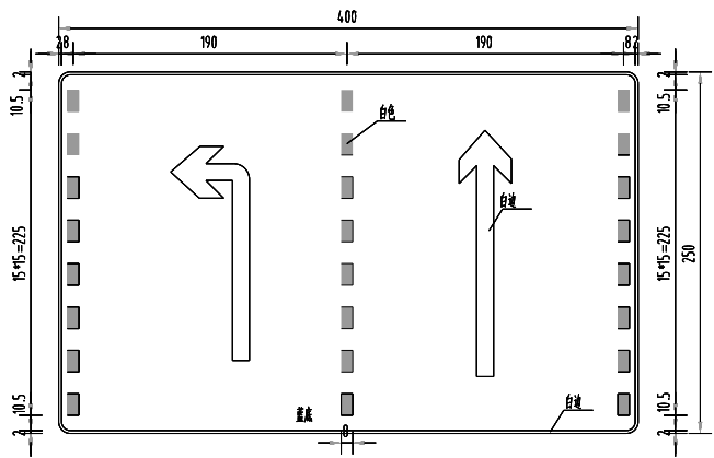
分车道行驶标志版面尺寸
