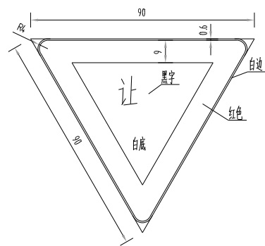
三角形禁令标志牌版面尺寸
