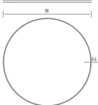
圆形指示标志牌版面尺寸
