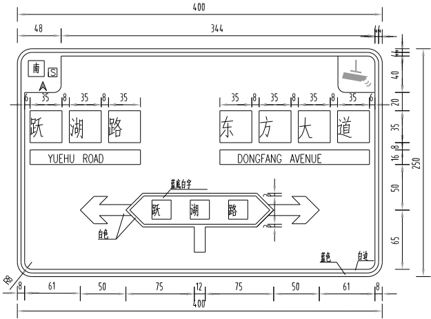
交叉口指路标志牌版面尺寸
