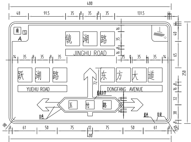
交叉口指路标志牌版面尺寸
