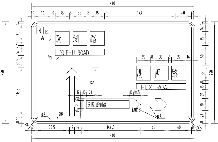
交叉口指路标志牌版面尺寸
