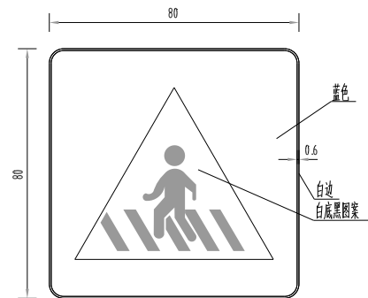
正方形指示标志牌版面
