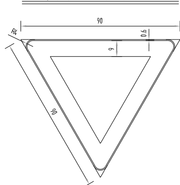
三角形禁令标志牌版面尺寸
