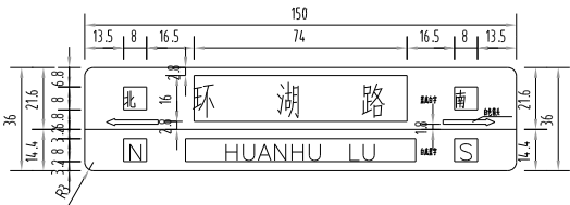
路名牌标志版面尺寸
