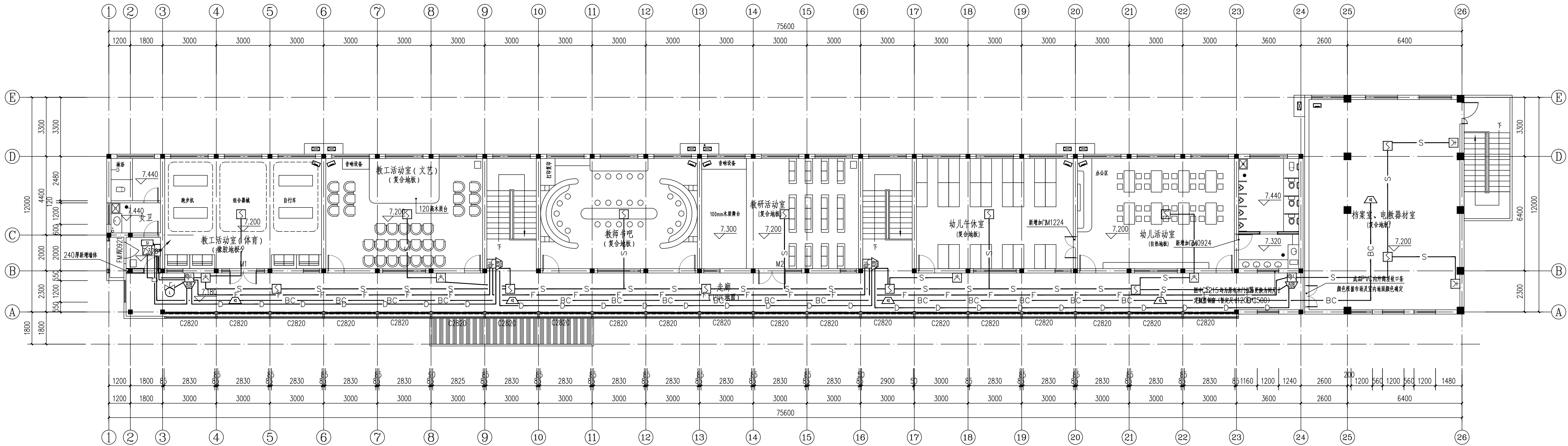
三层火灾自动报警平面图 1:100
