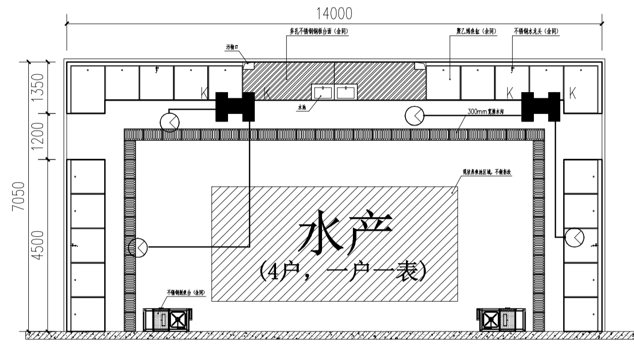
水产摊位平面图 1:50
