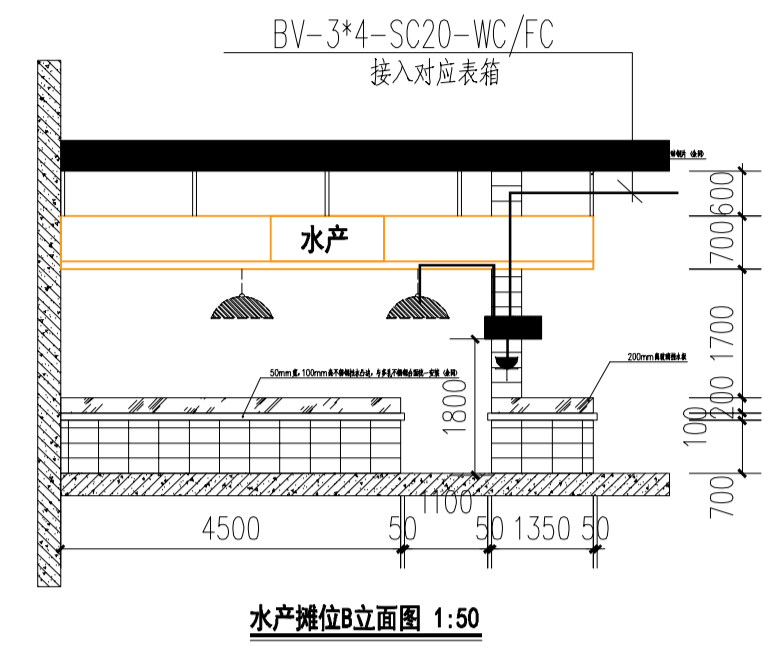
水产摊位立面图 1:50
