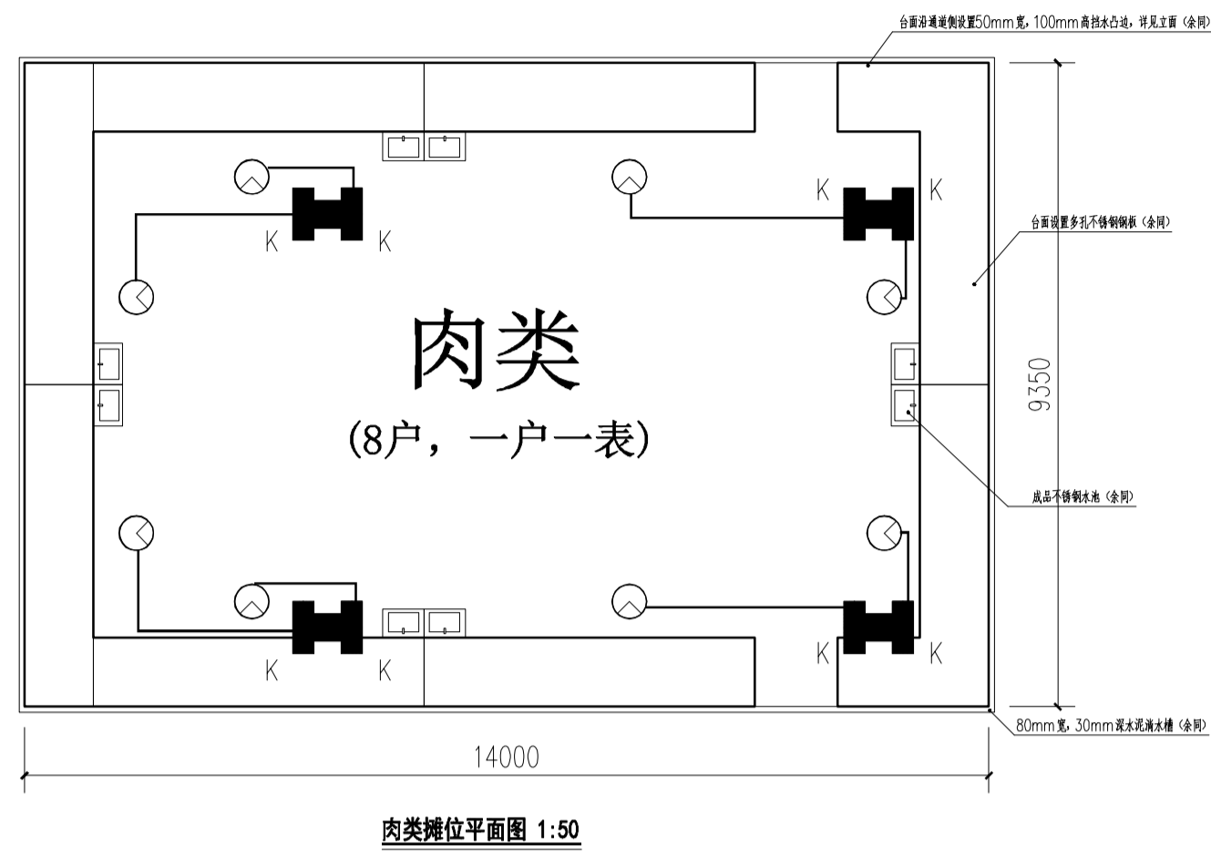
肉类摊位平面图 1:50
