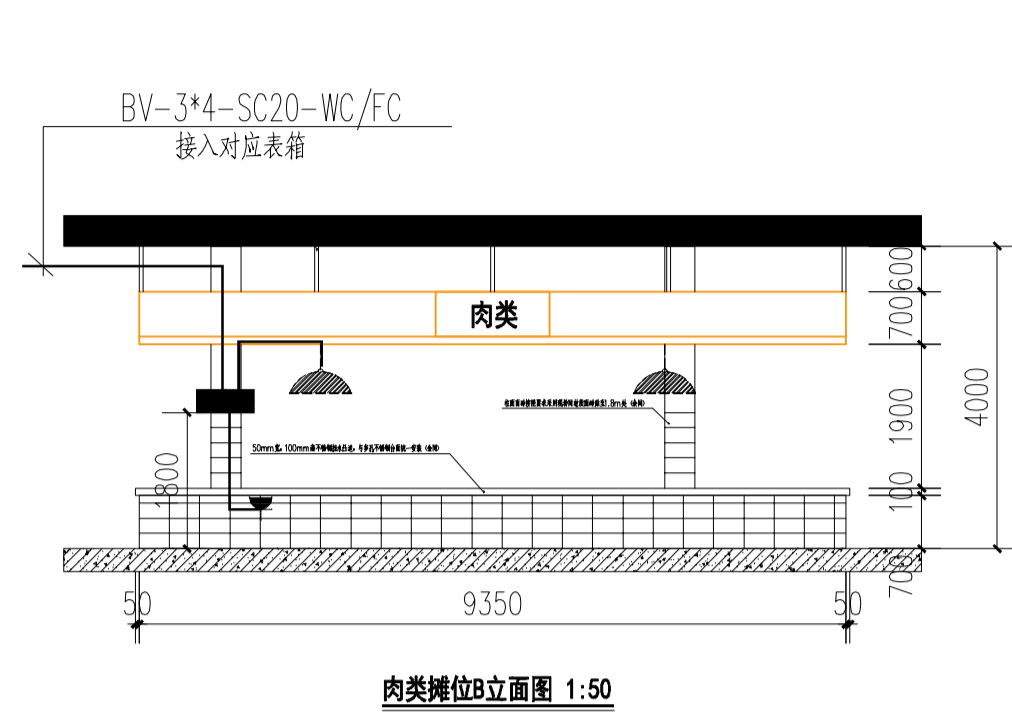
肉类摊位立面图 1:50
