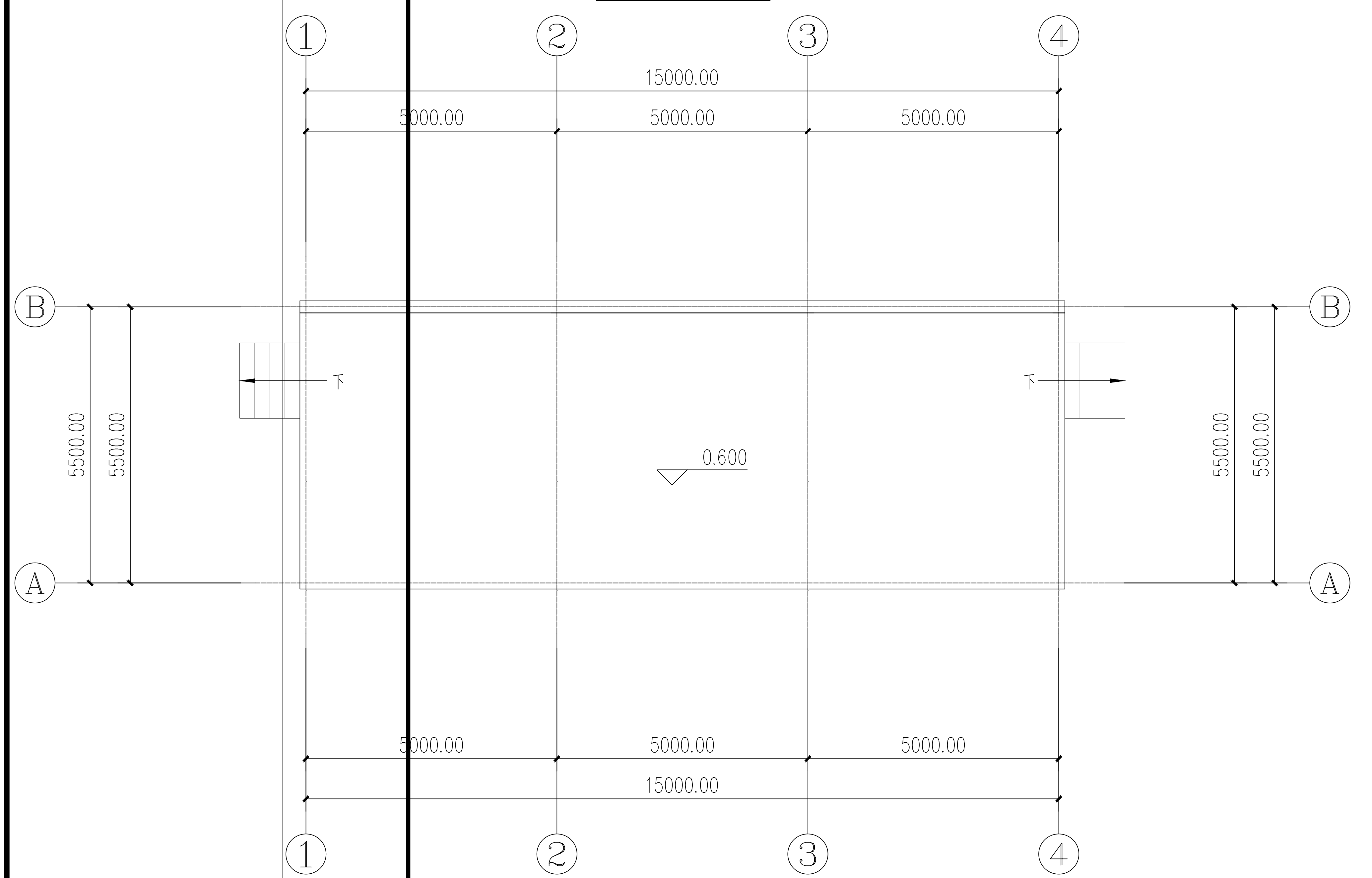
屋顶层平面图 1:100
