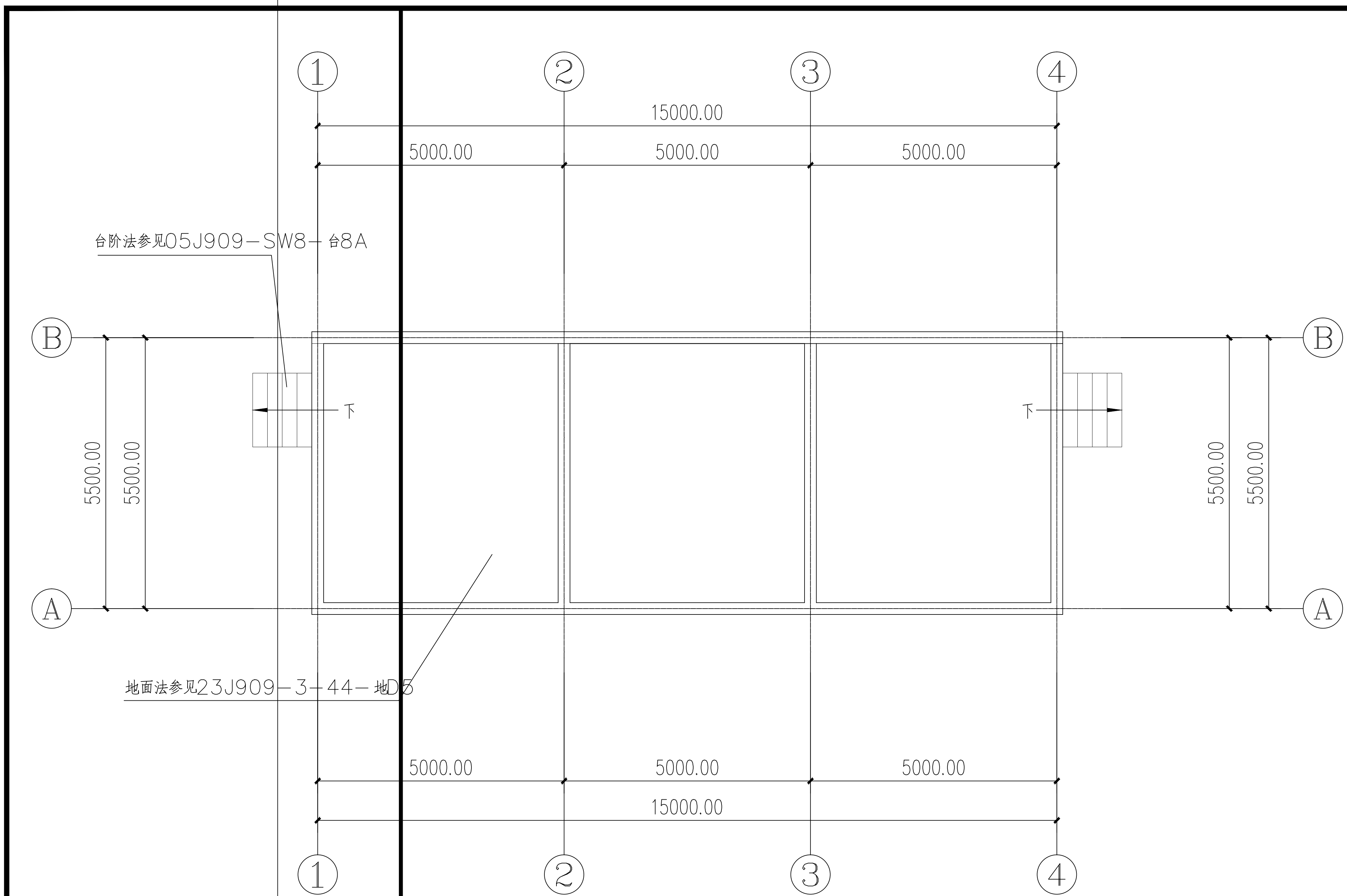
一层平面图 1:100
