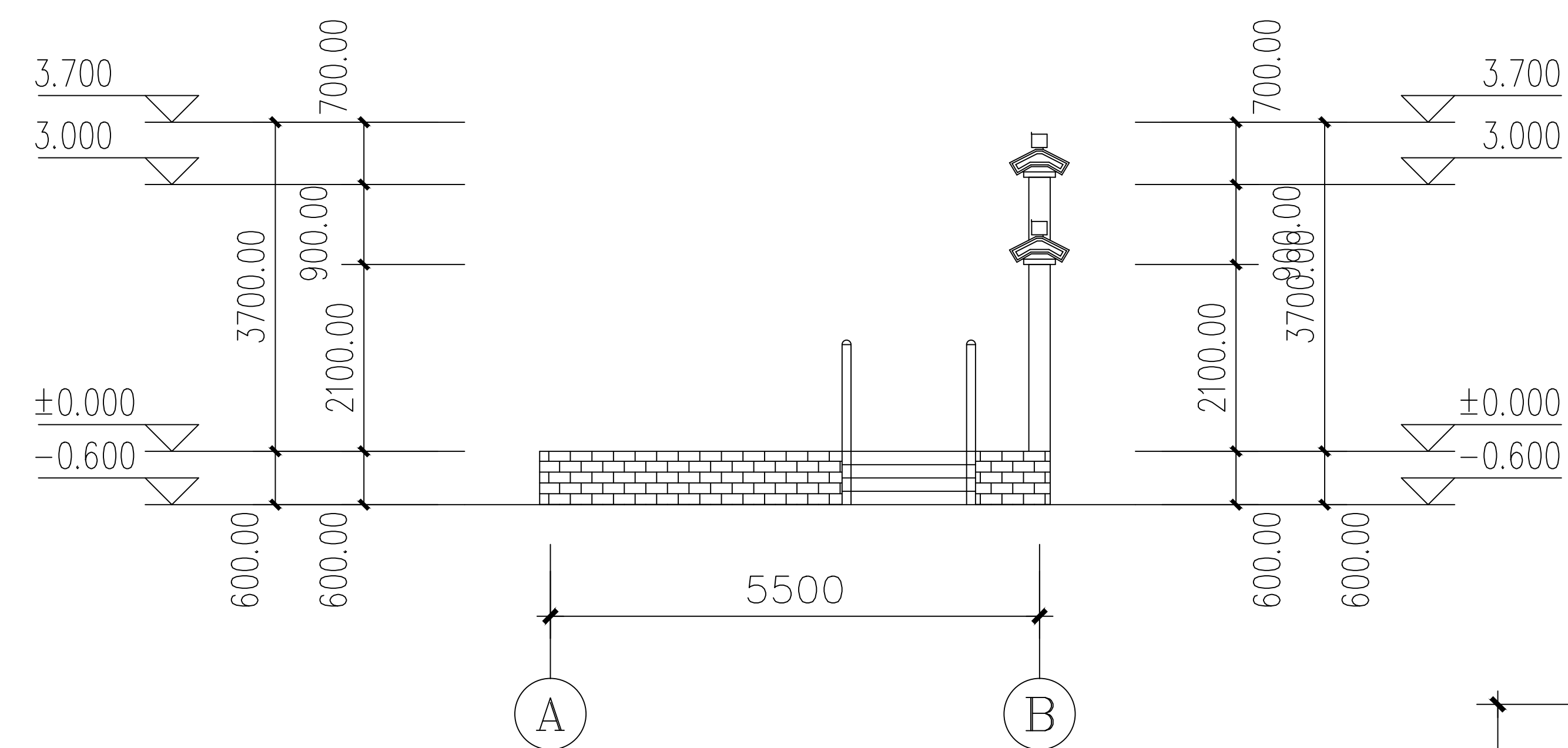
①—④立面图 1:100
