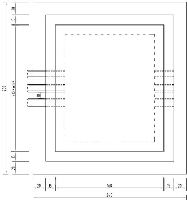
交叉口过路管线套管检查井平面
