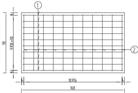
检查井盖平面图
