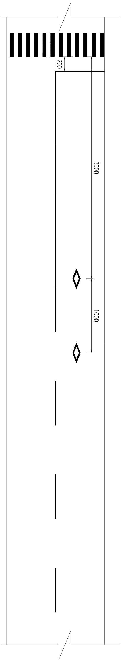
人行道标线布置图
