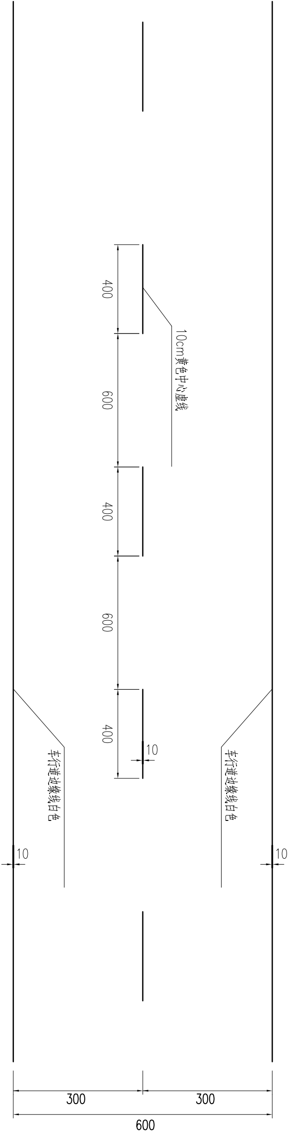
路面标线布置大样图
