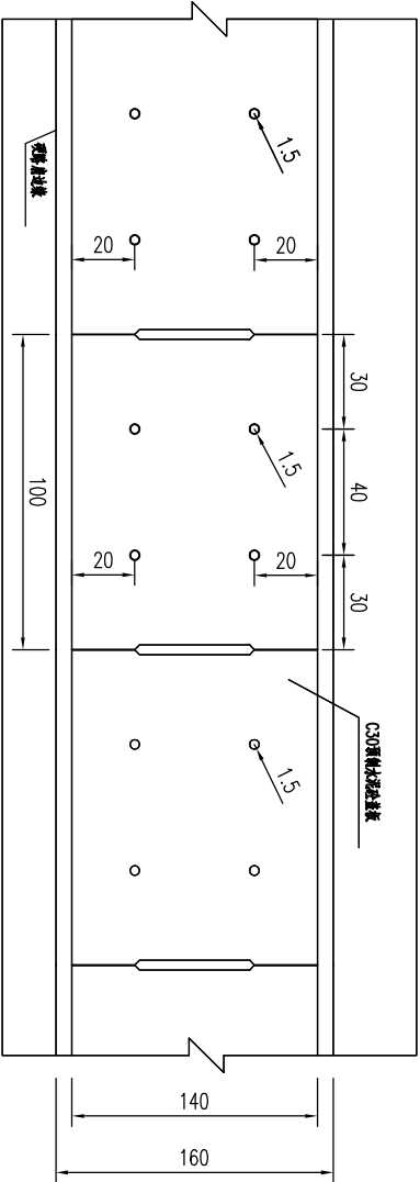
排水方沟平面布置图
