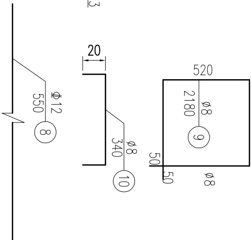
基础锚板平面
