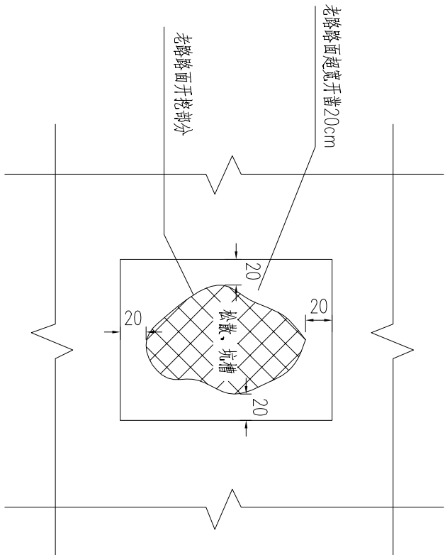
水泥砼板板角损坏处理示意图
