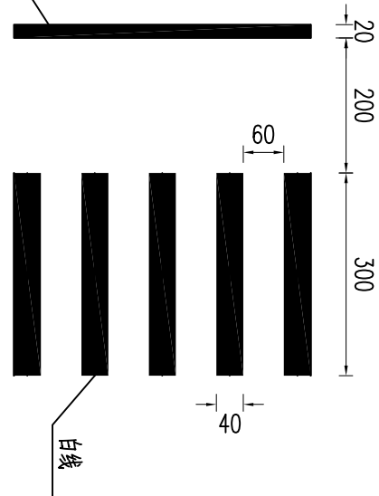
人行横道（正交）
