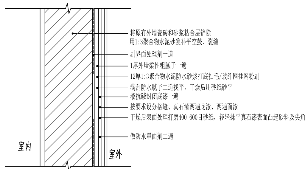
外墙真石漆做法 1:10
