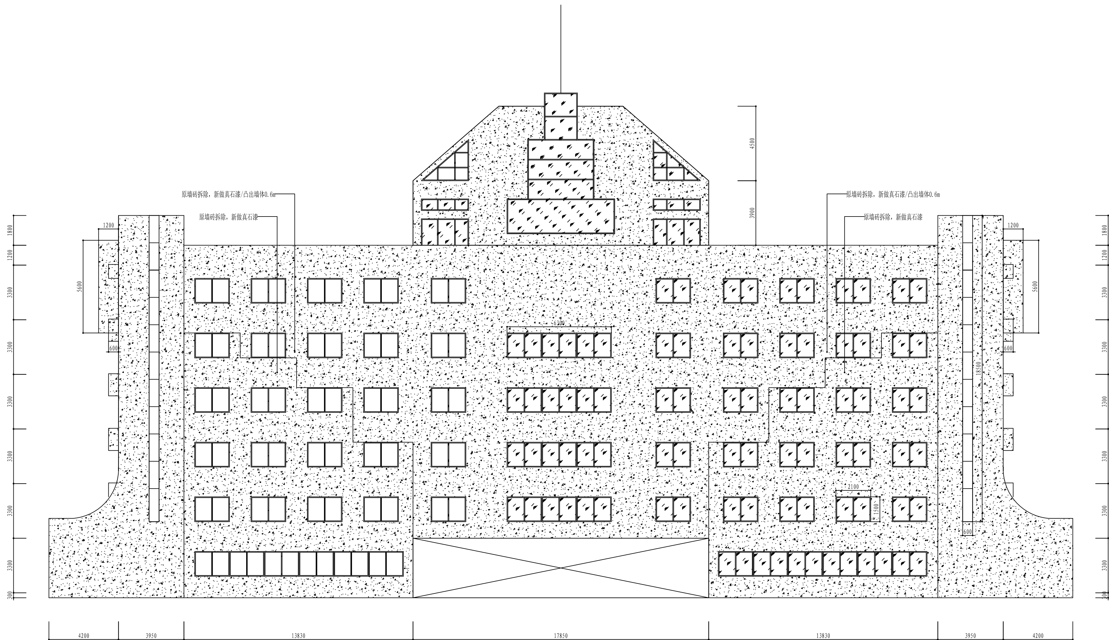
南立面图 1:100
