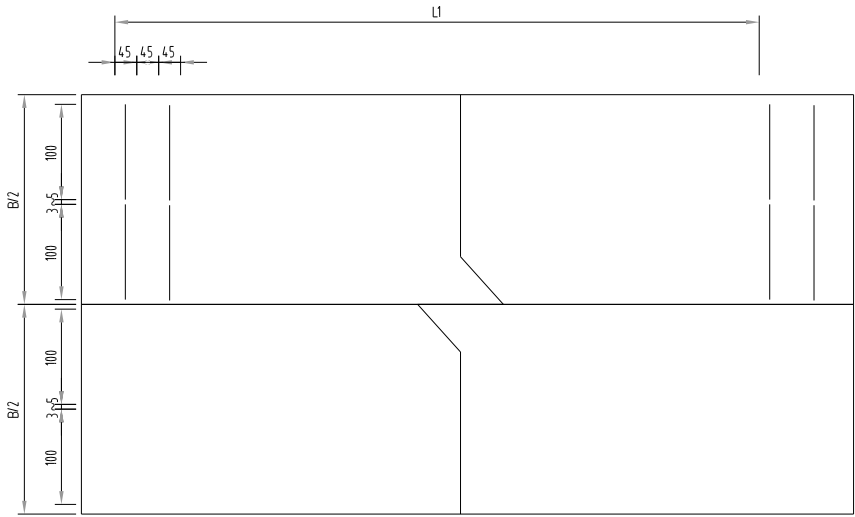
横向震荡标线布置图
