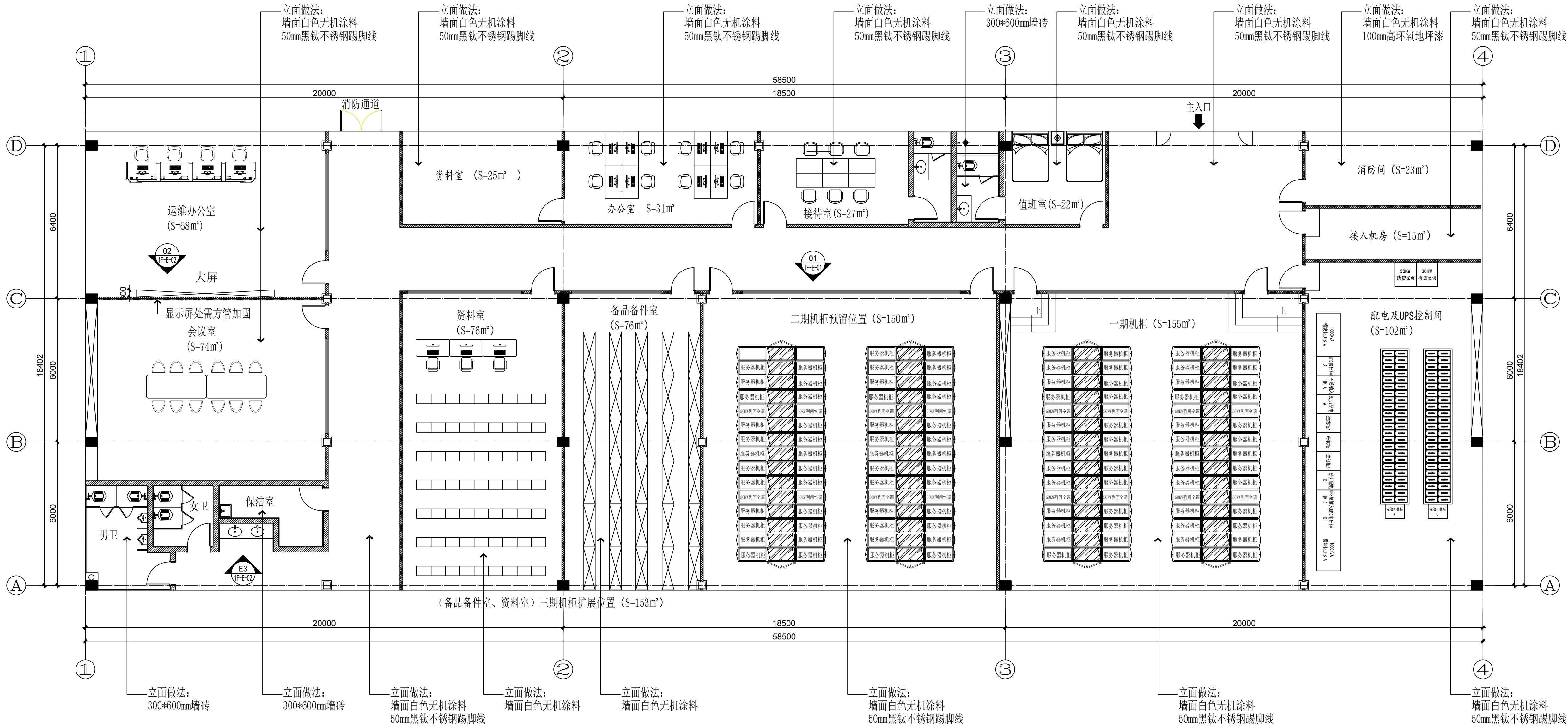
TOP PLAN 一层立面索引图 SCALE 1:100
