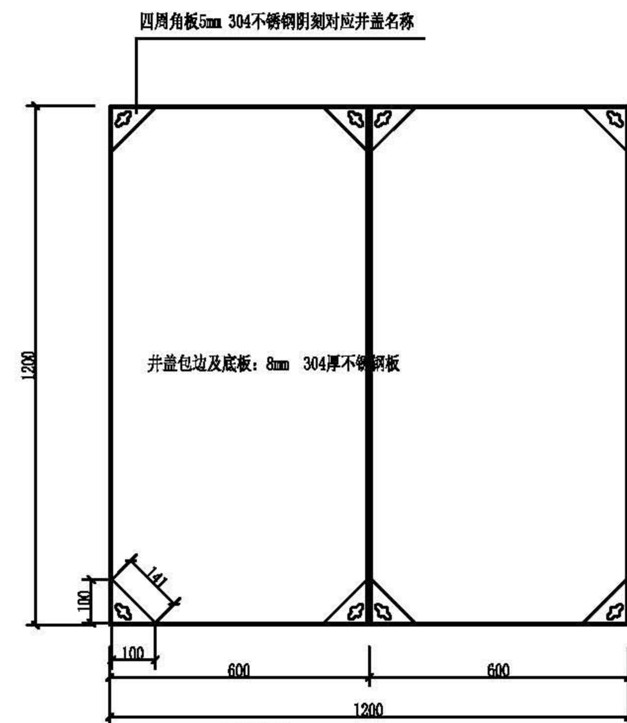
井盖平面图
