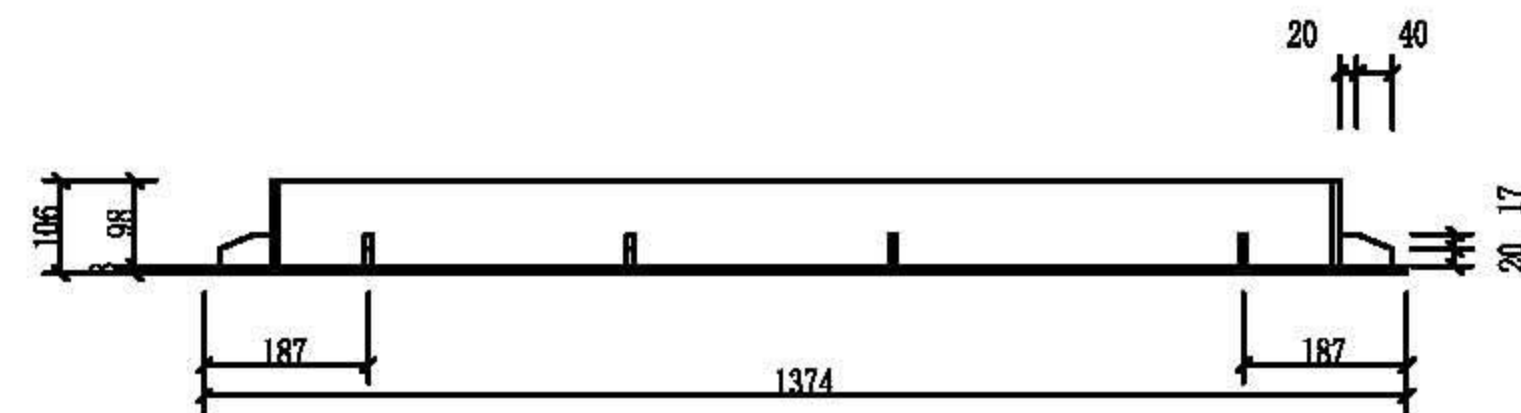
井框侧面图
