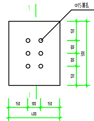
盖板平面
