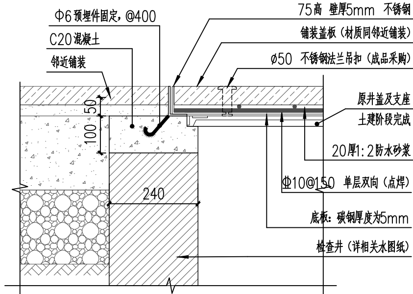
④ 车行道路 装饰井盖固定大样 1:10
