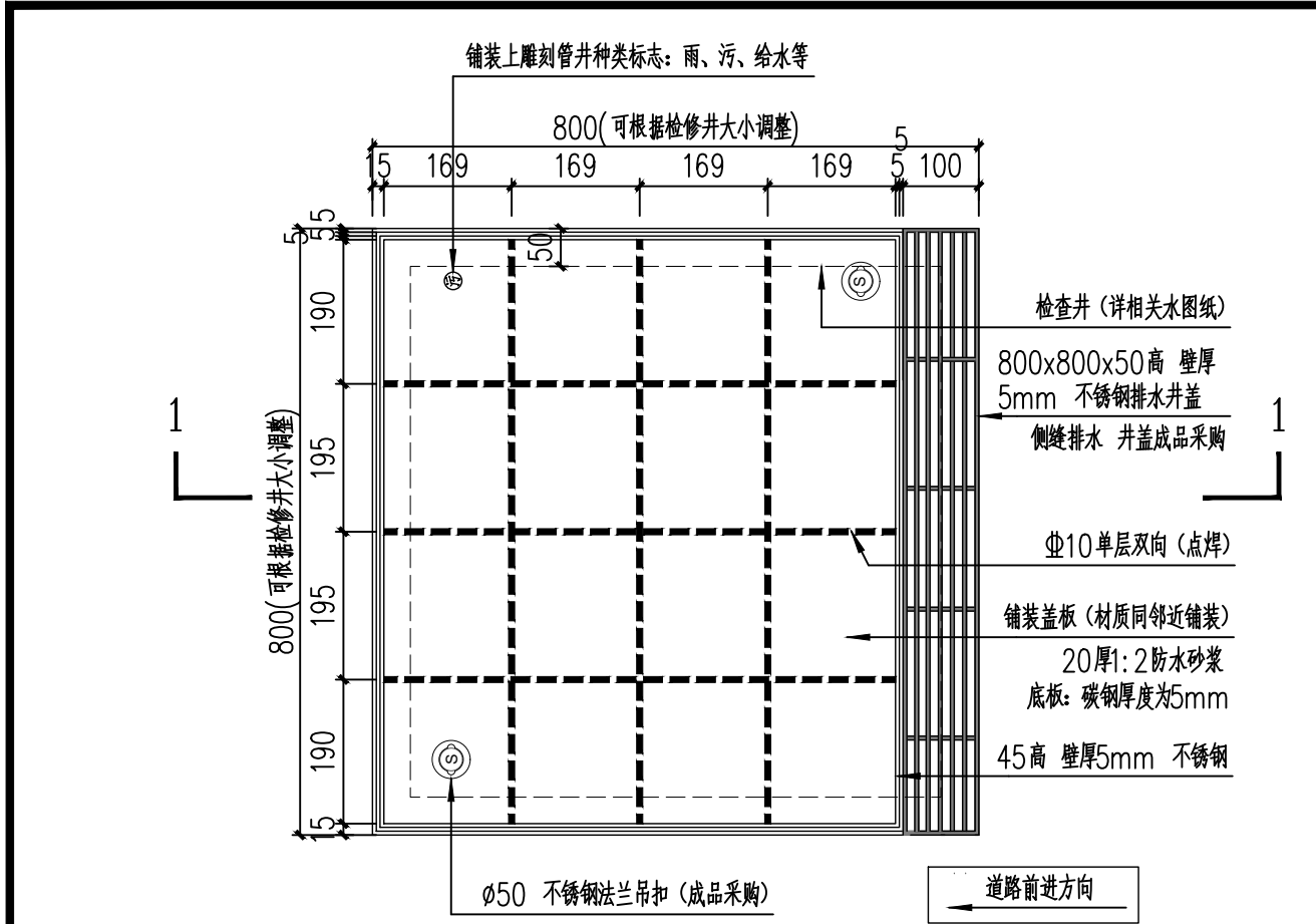
① 人行道路 装饰井盖平面 1:10
