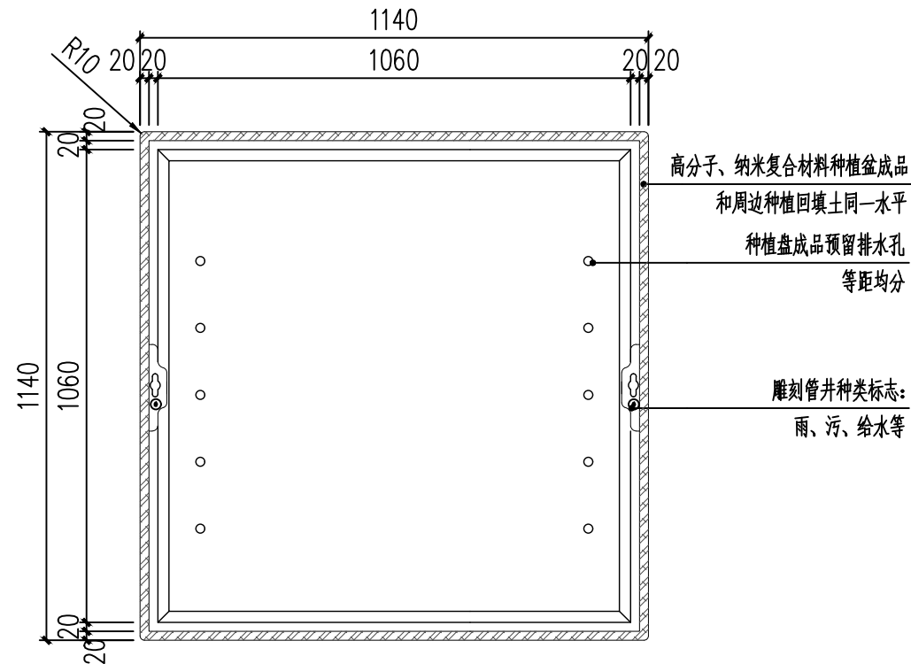
⑥ 绿化种植盆平面图 1:15
