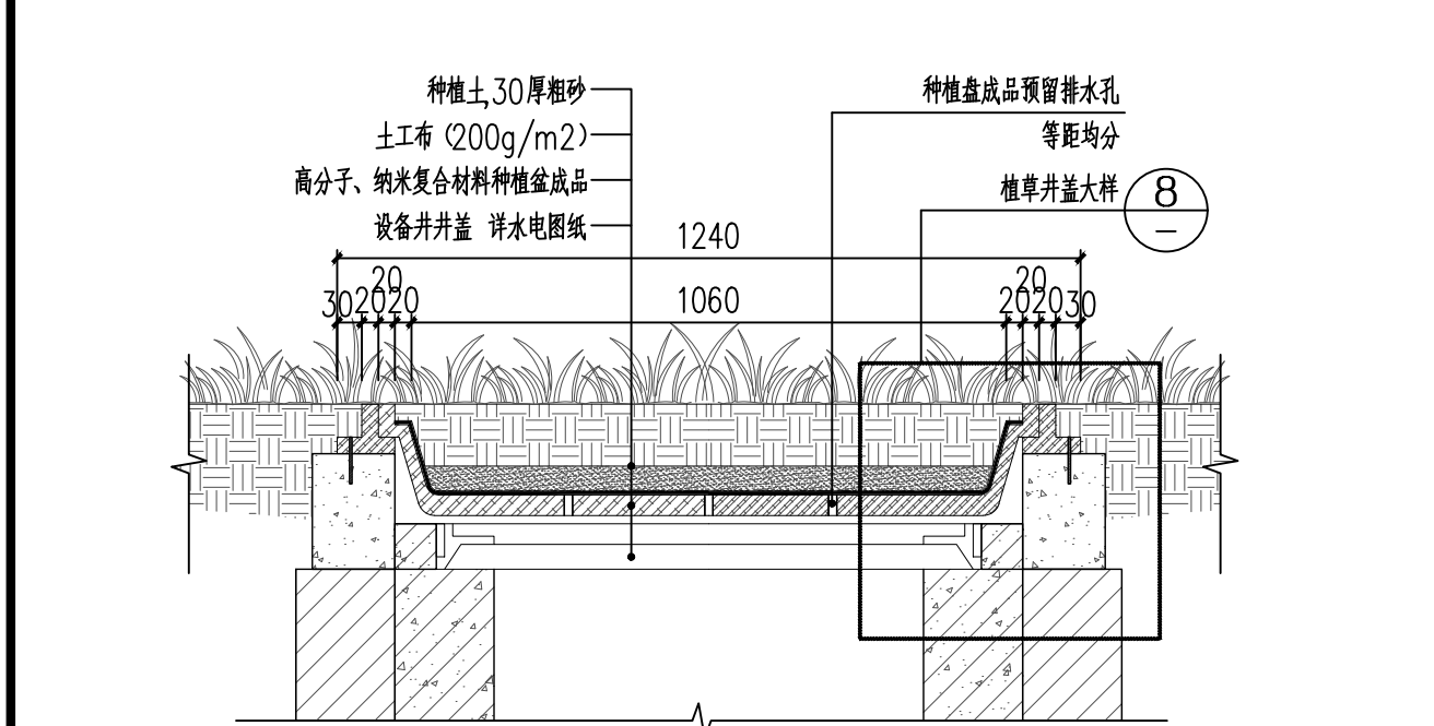
⑦ 植草井盖剖面做法 1:10
