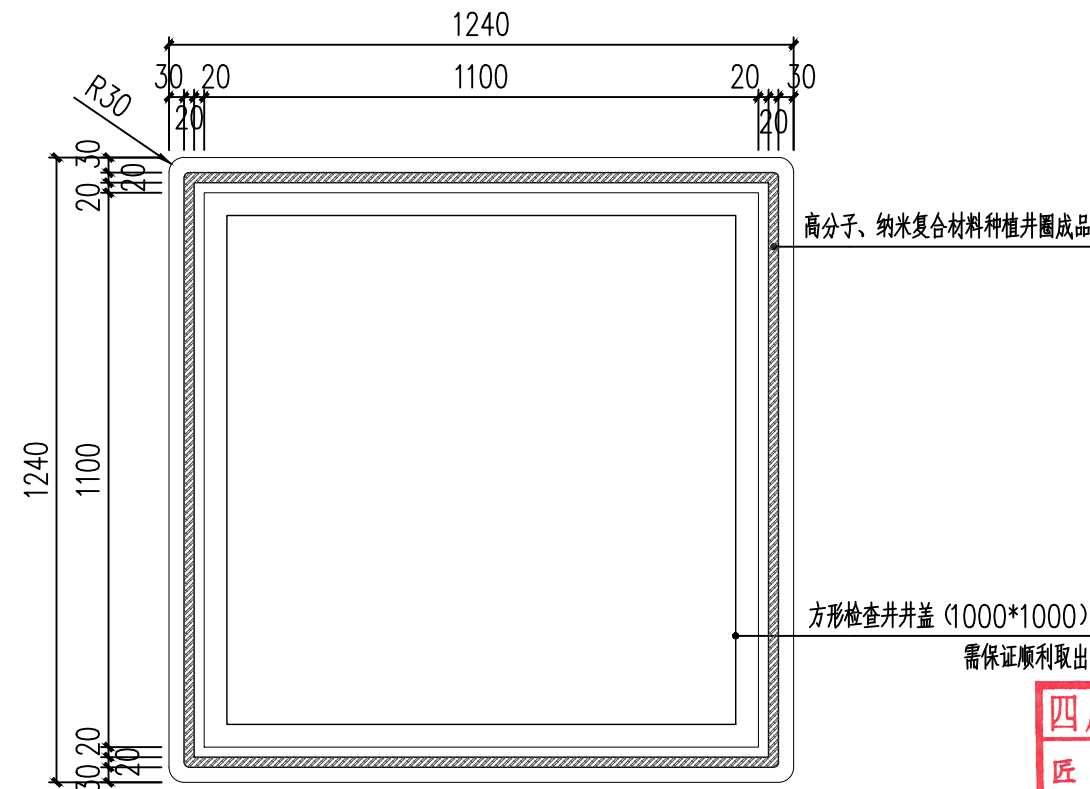
⑤ 绿化种植井圈平面图 1:15
