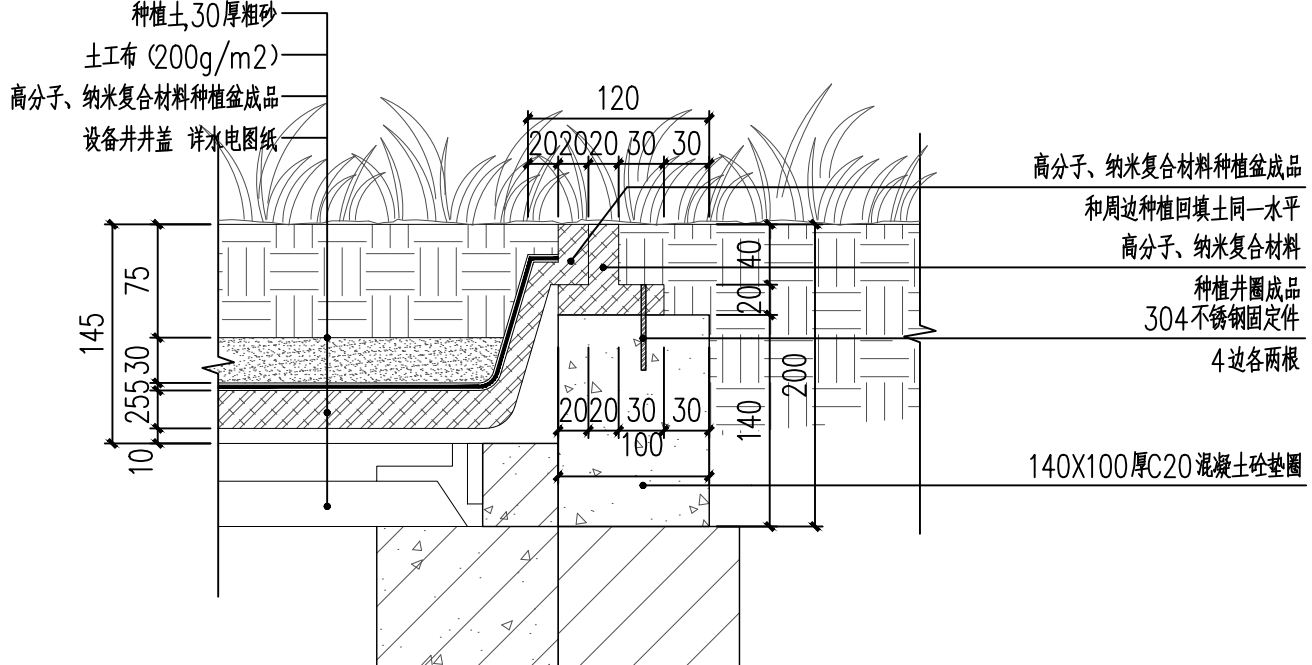
⑧ 植草井盖大样 1:5
