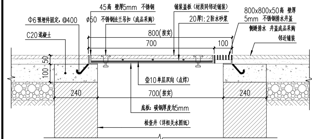
② 人行道路 1-1 剖面图 1:10
