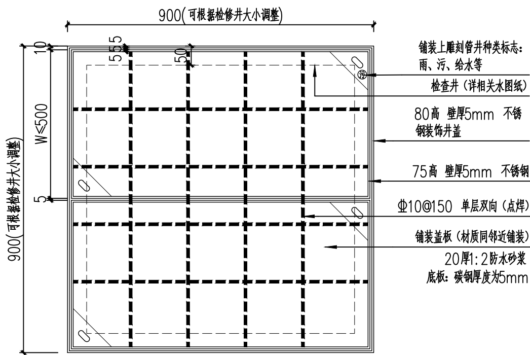
③ 车行道路 装饰井盖平面 1:10
