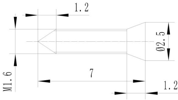
图 59a 领花结构和主要尺寸
