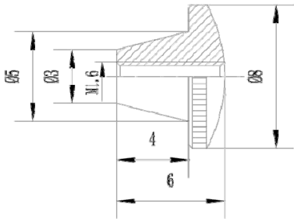
图 59b 螺钉结构及主要尺寸
