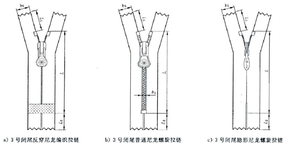
图 75 尼龙拉链
