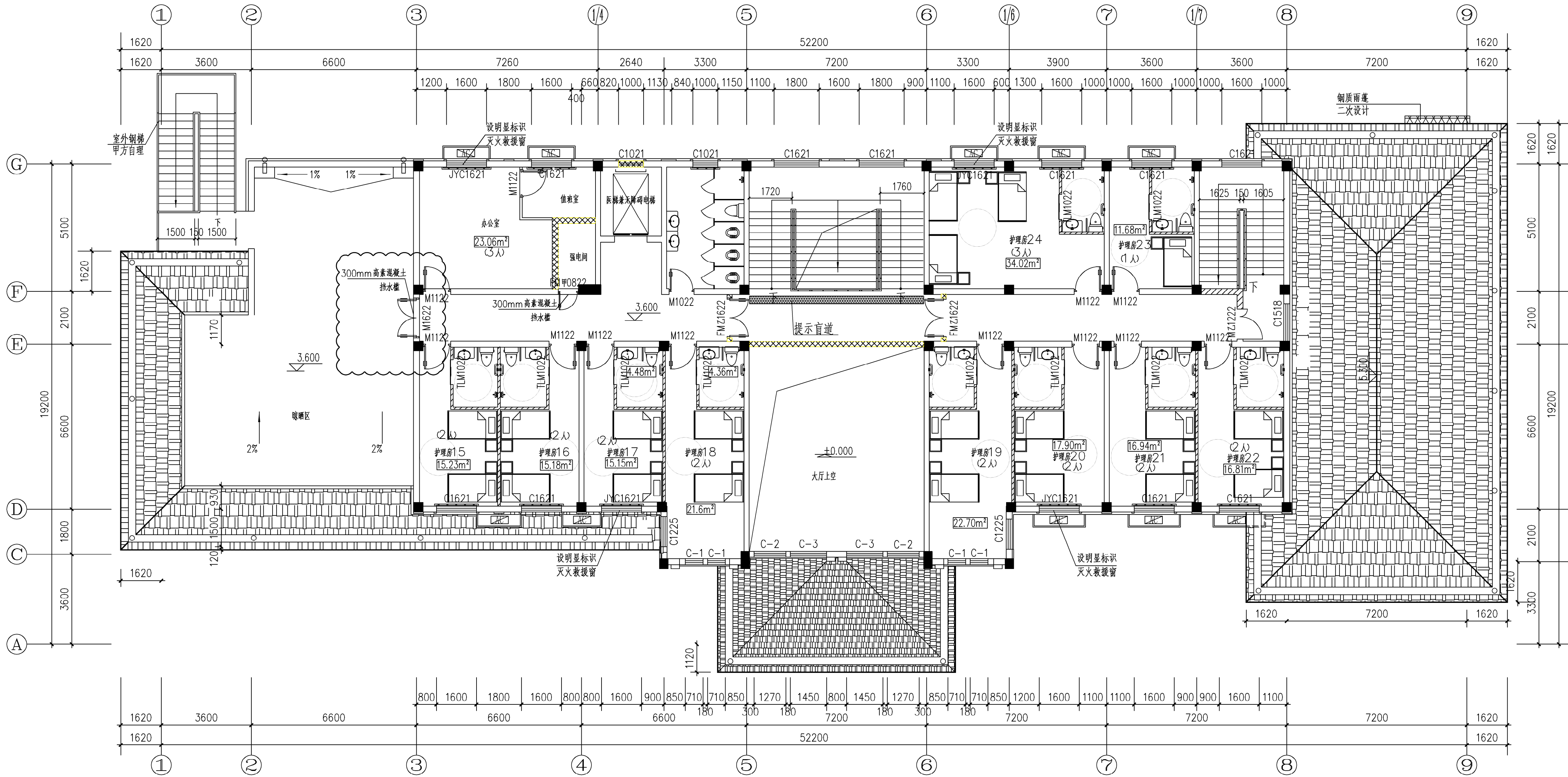
二层消防报审平面图 1:100
