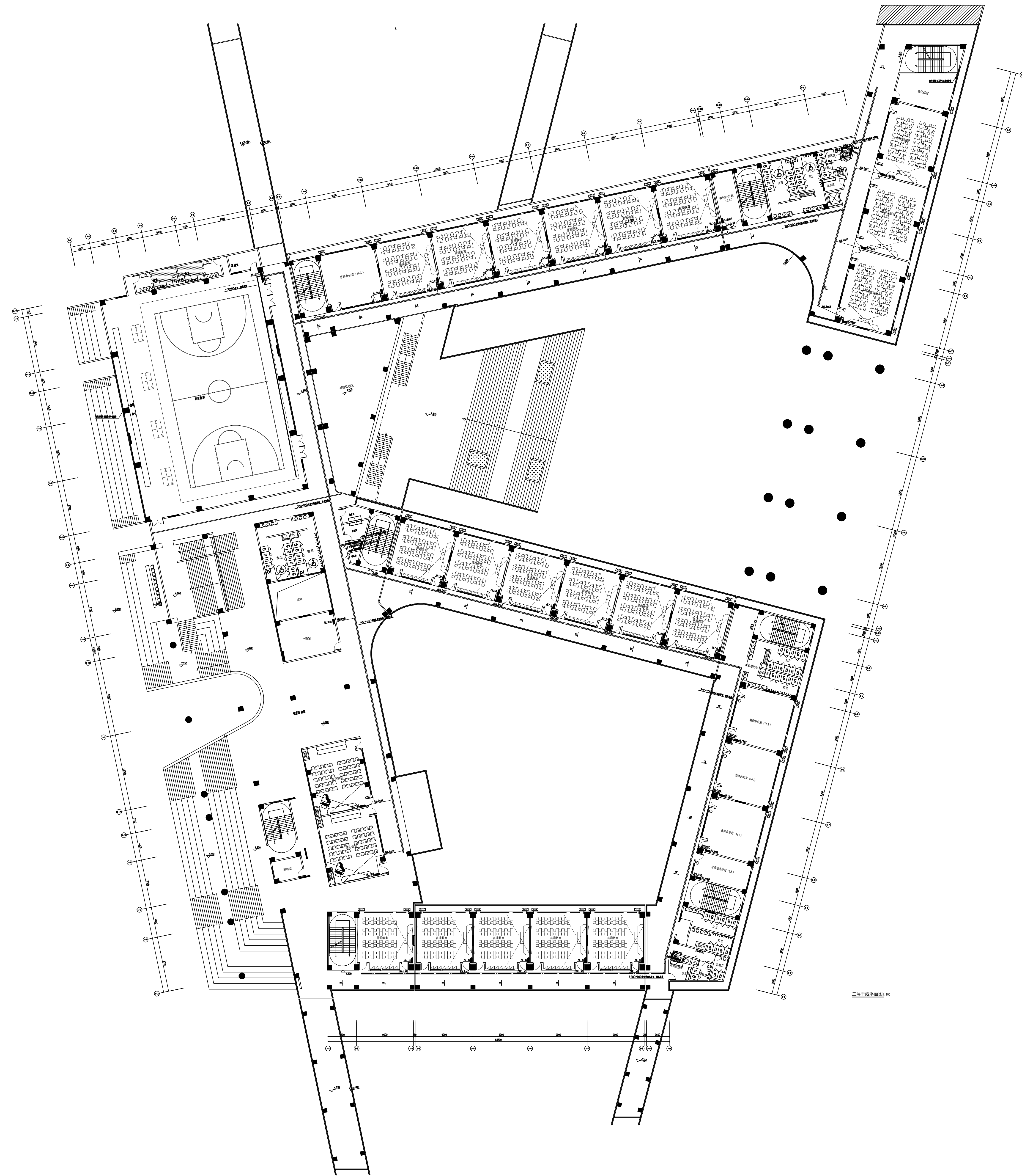
教学楼二层
