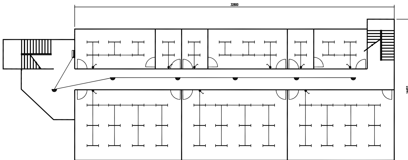
一层~五层平面示意图 1:100
