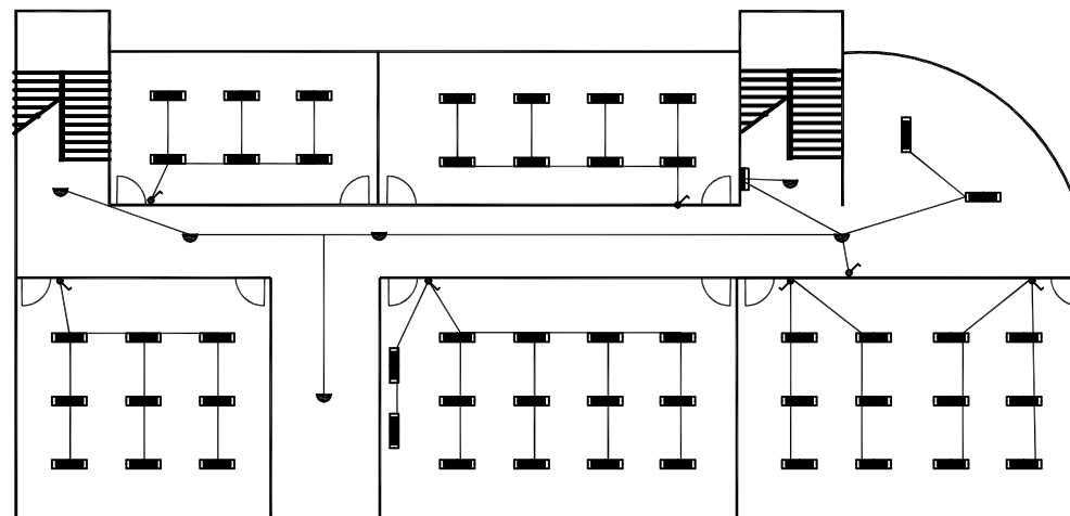
一层局部平面示意图 1:100
