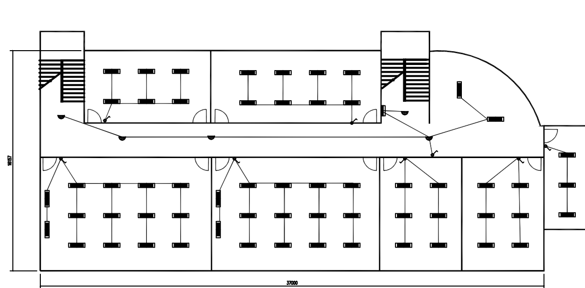
二~五层平面示意图 1:100
