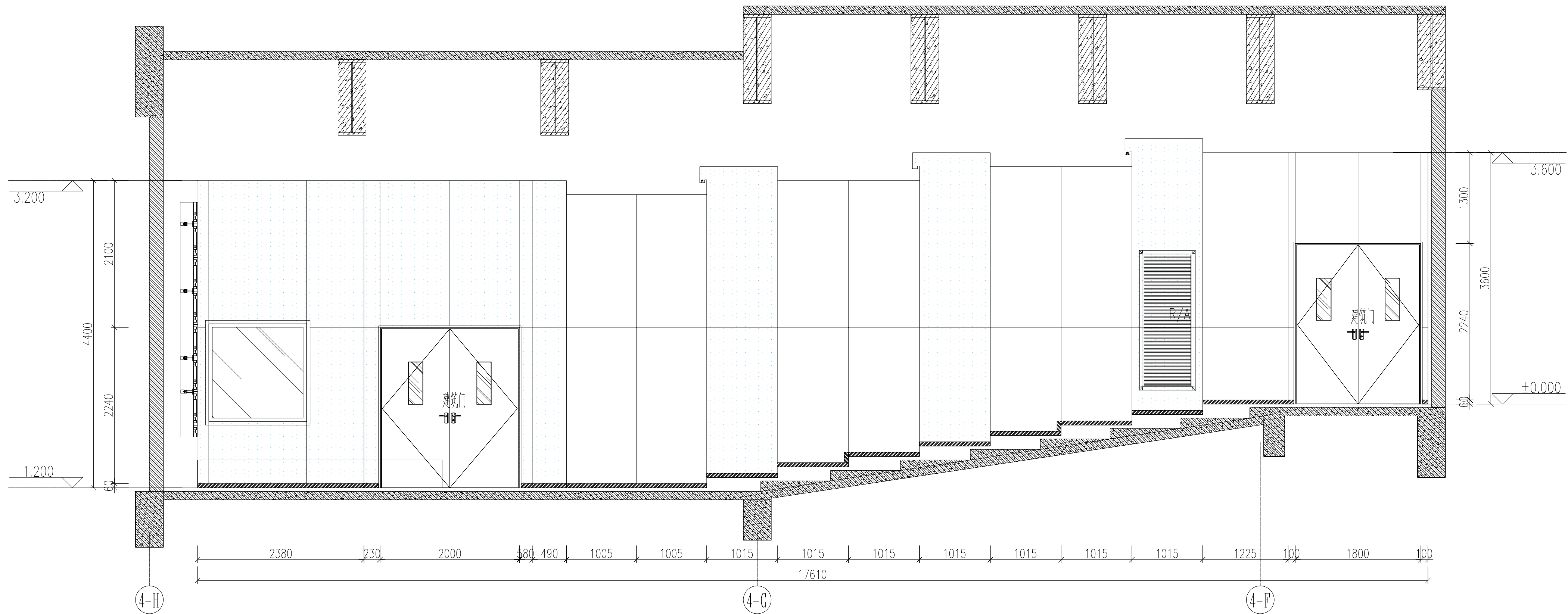
国际交流中心 1F报告厅剖面
