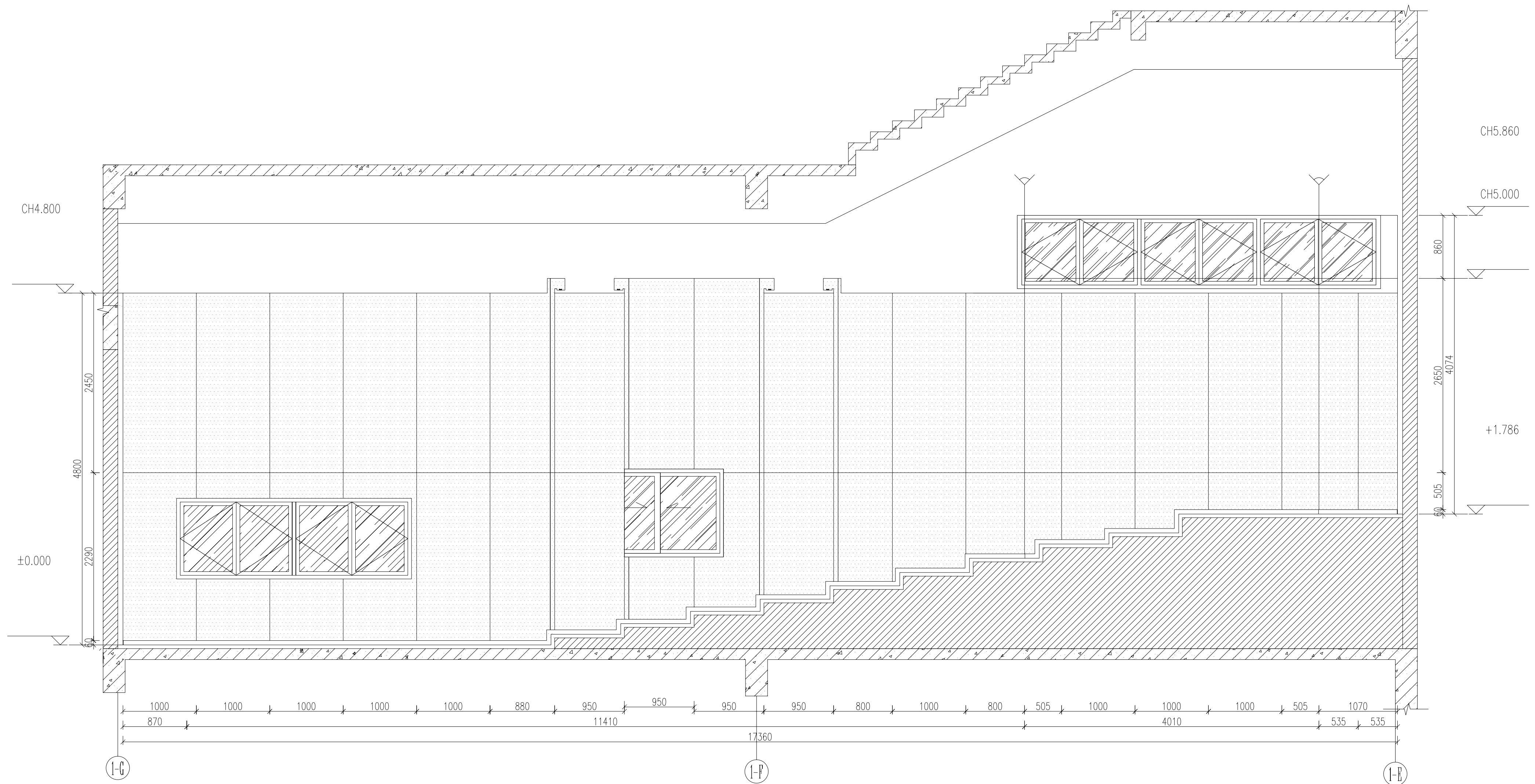
A区一层1F报告 厅剖面
