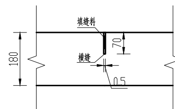
横向缩缝构造图
