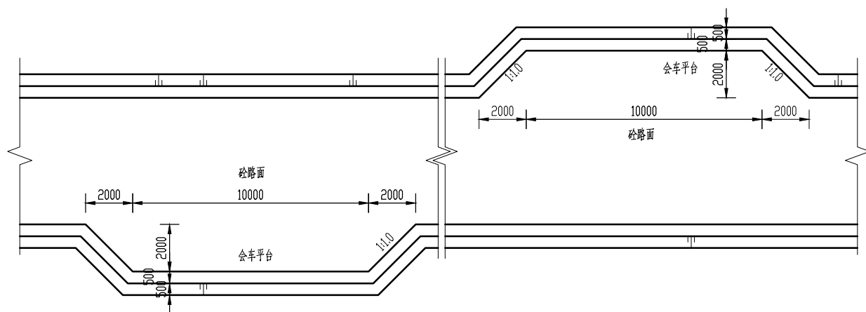
会车平台示意图
