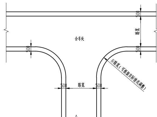
道路交汇处示意图
