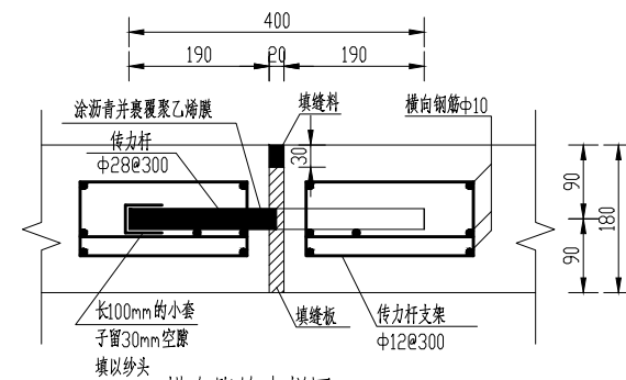
横向胀缝大样图
