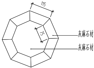
路牌平面图 1:5
