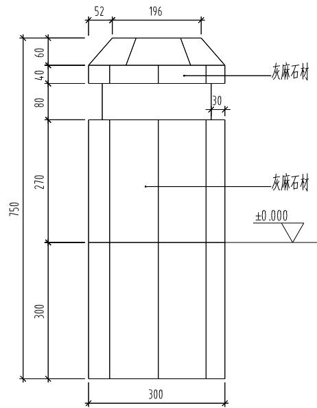
路牌立面图 1:5
