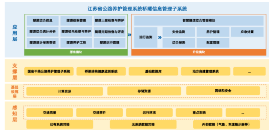
图 10-1 总体架构图
