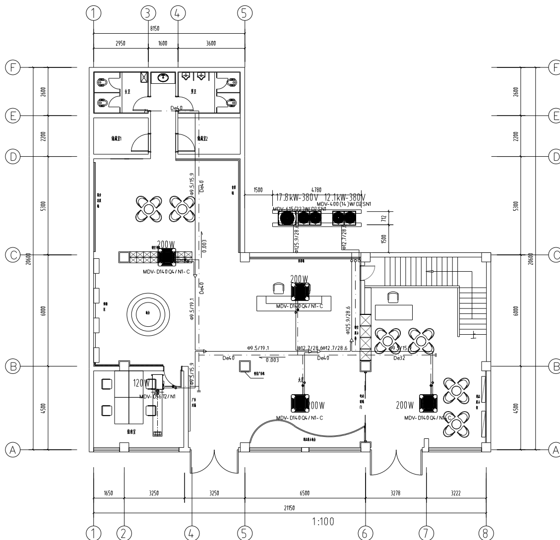
一层空调平面图 1:100
