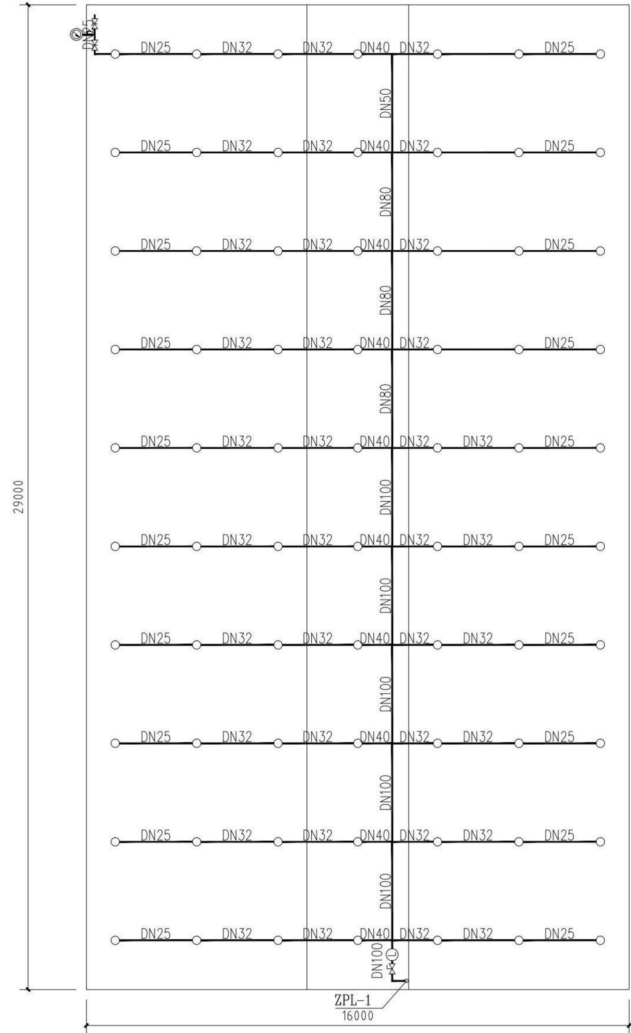
男生宿舍二至三楼喷淋布置平面图
