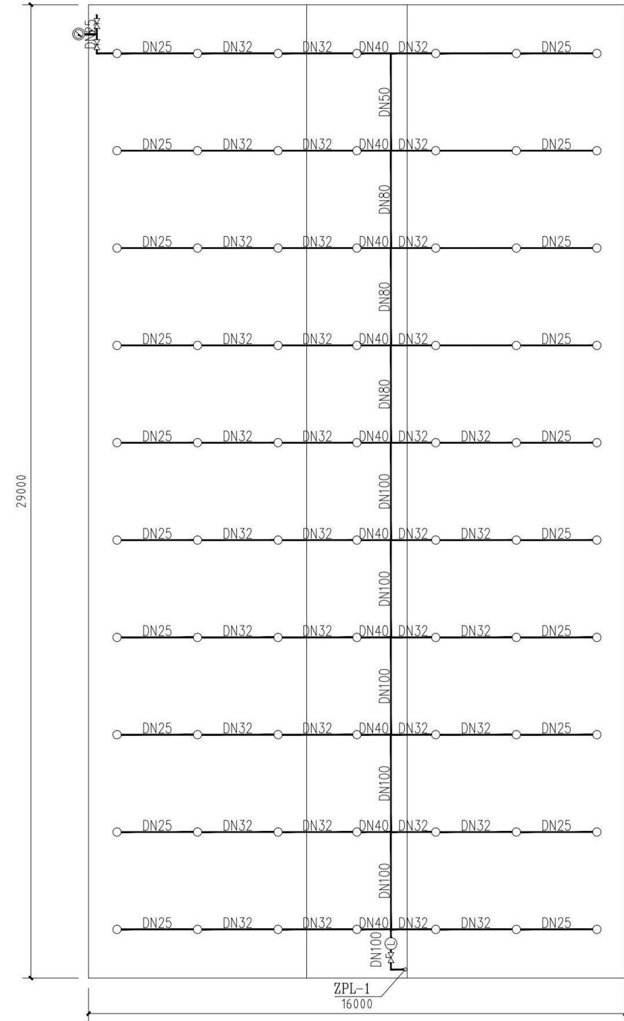
女生宿舍二至三楼喷淋平面布置图
