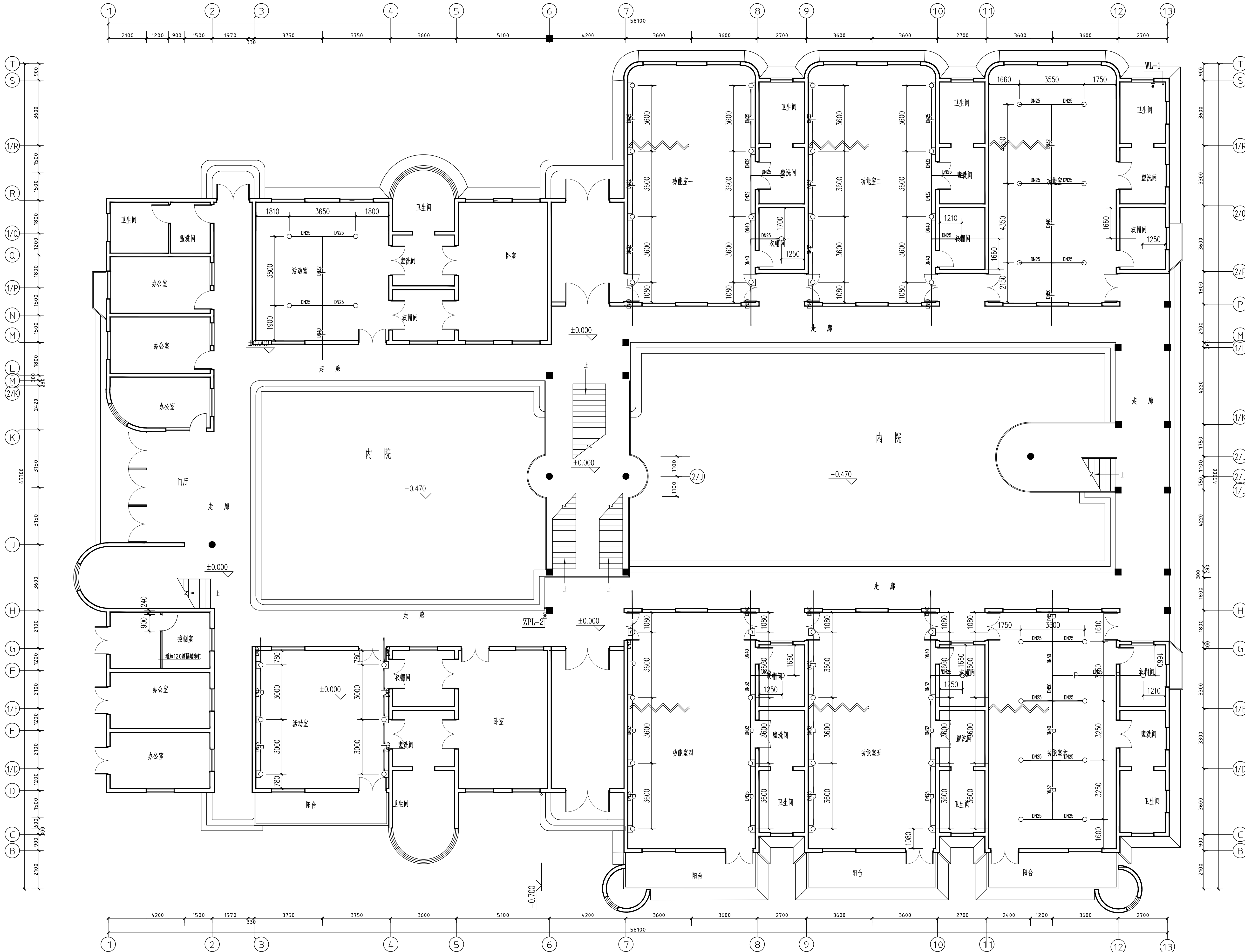
底层喷淋平面图 1:100
