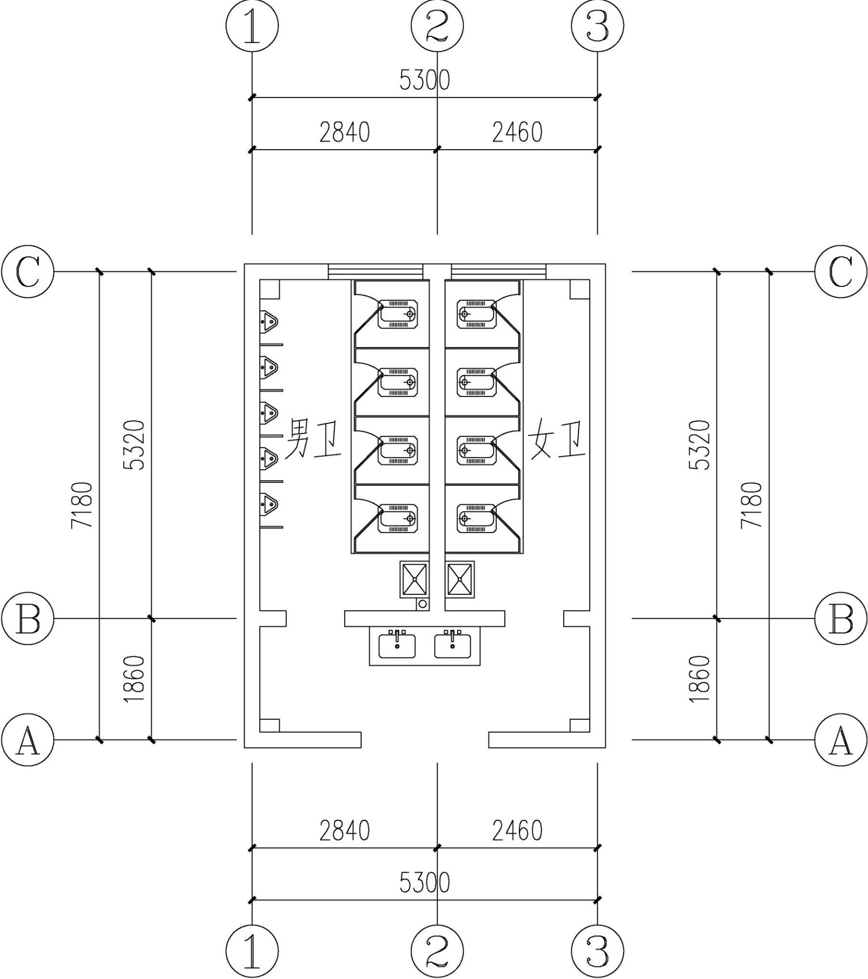
卫生间改造后平面图
