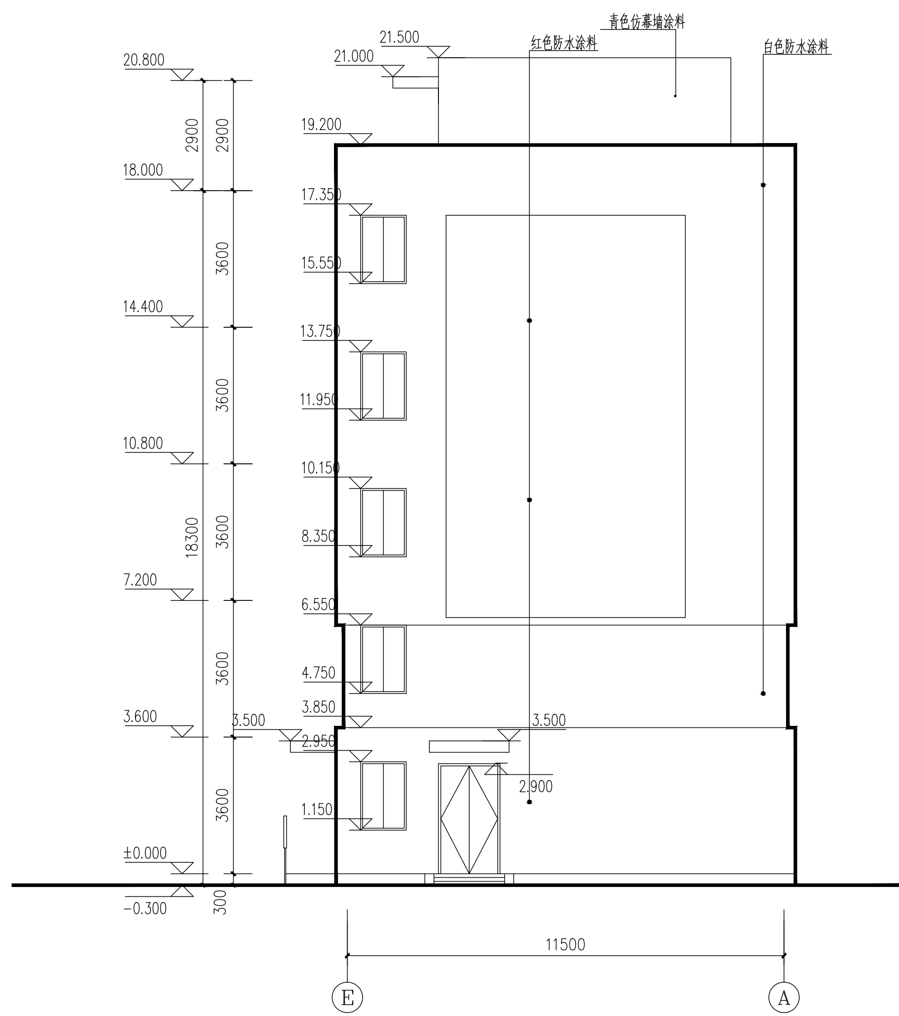
梦德轩宿舍楼西立面图100
