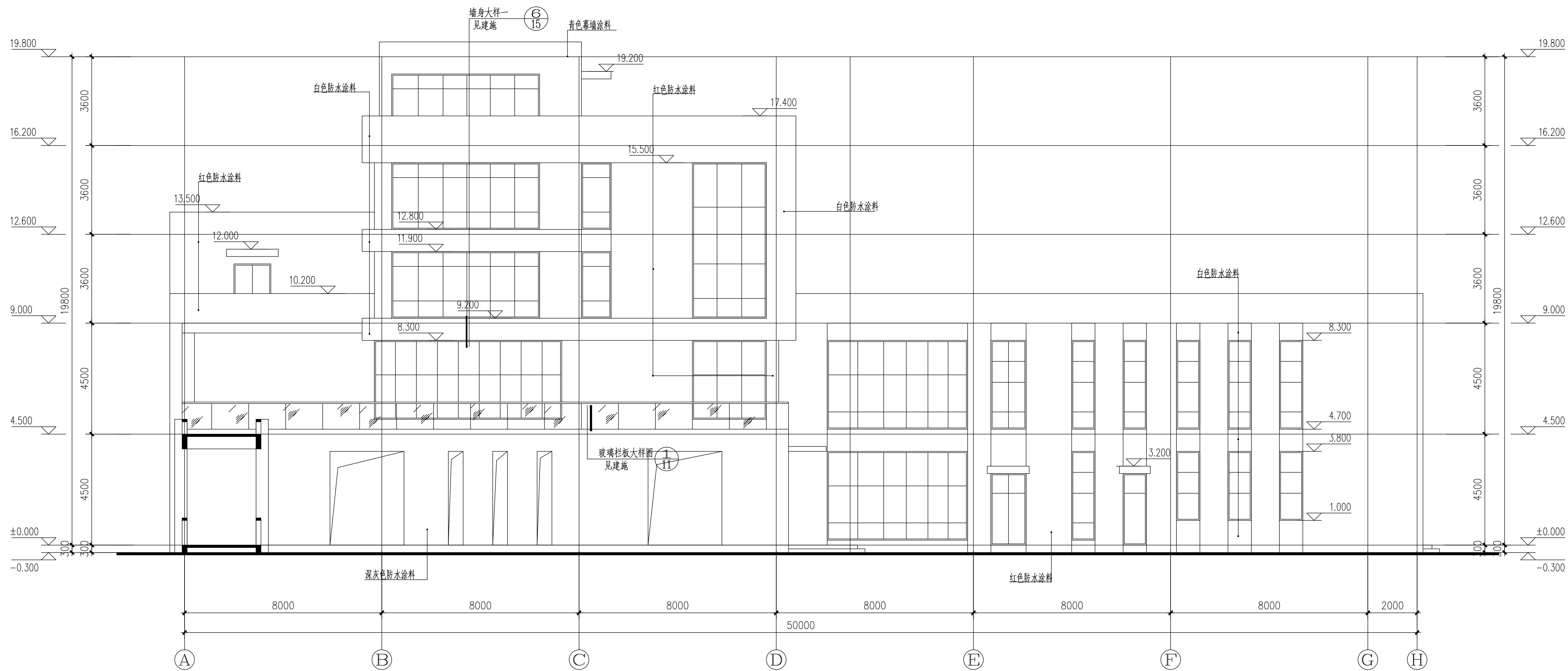
易安居东立面图:125
