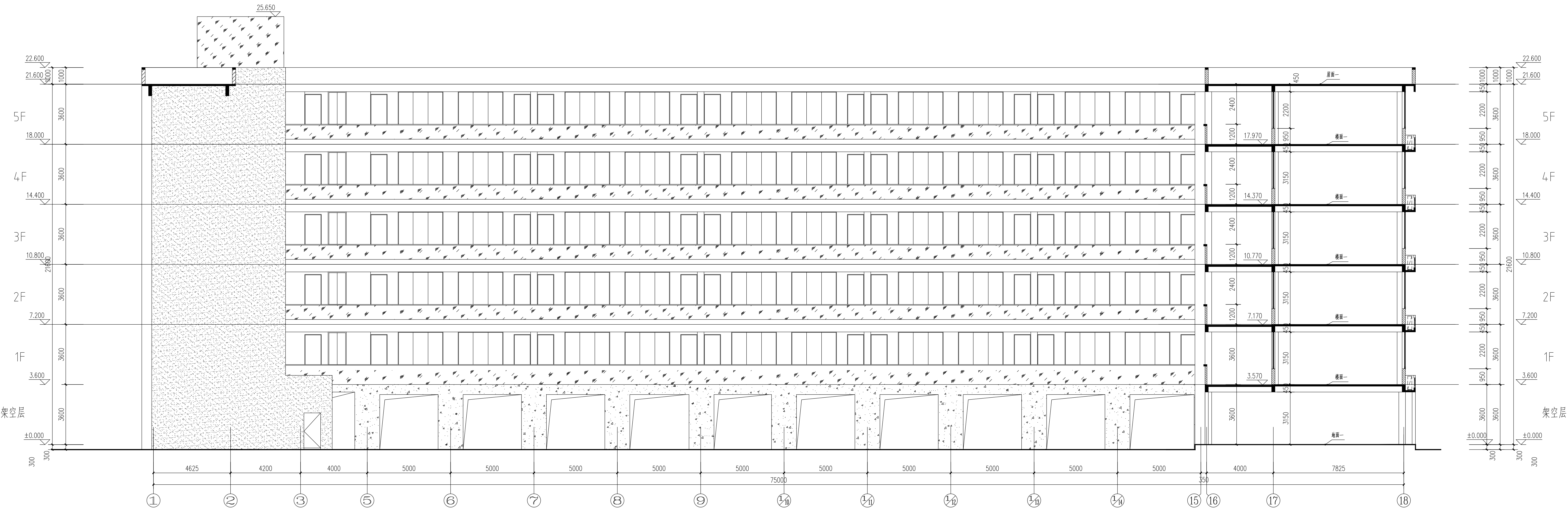
崇勇楼南立面图:200
