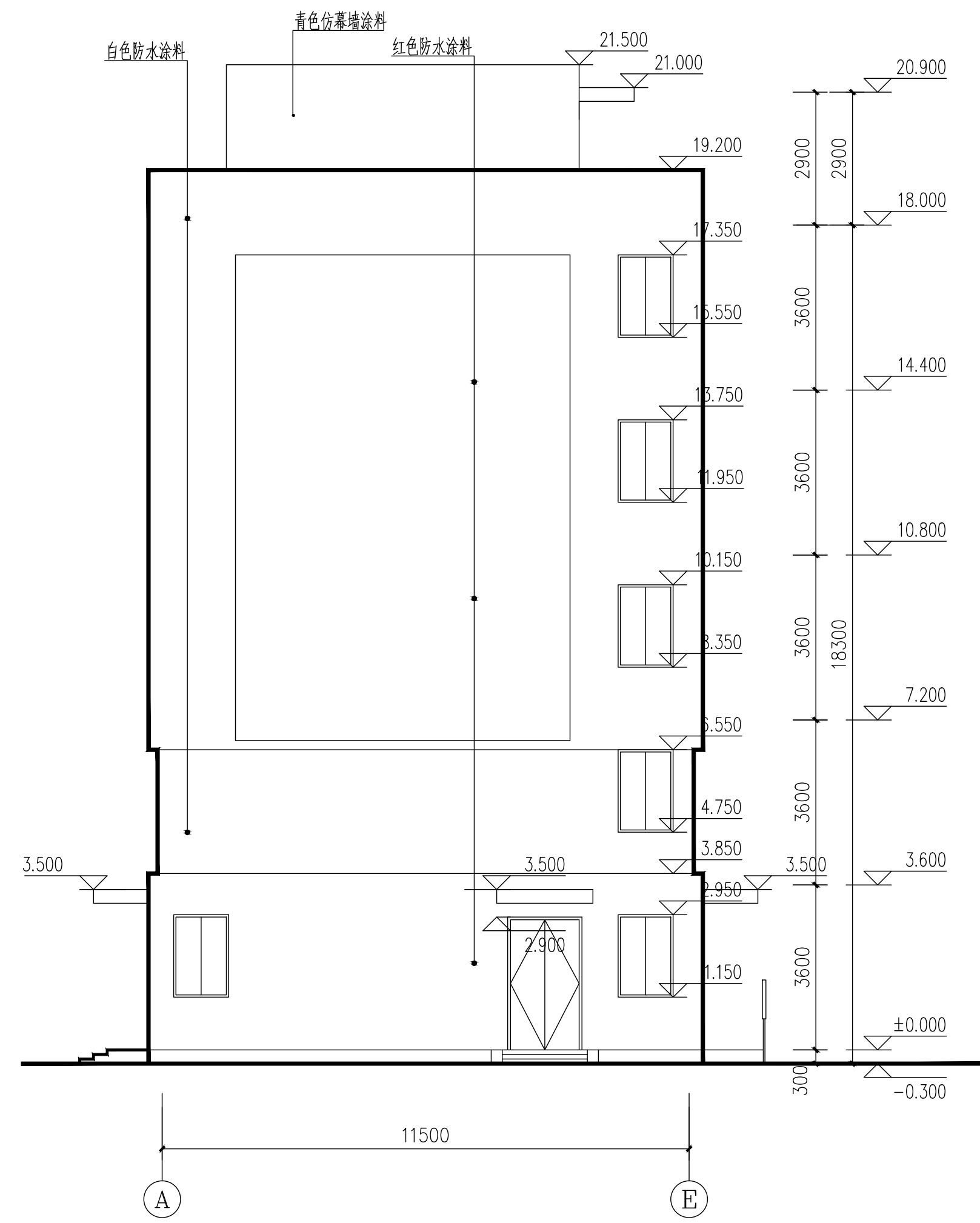
梦德轩宿舍楼东立面图100
