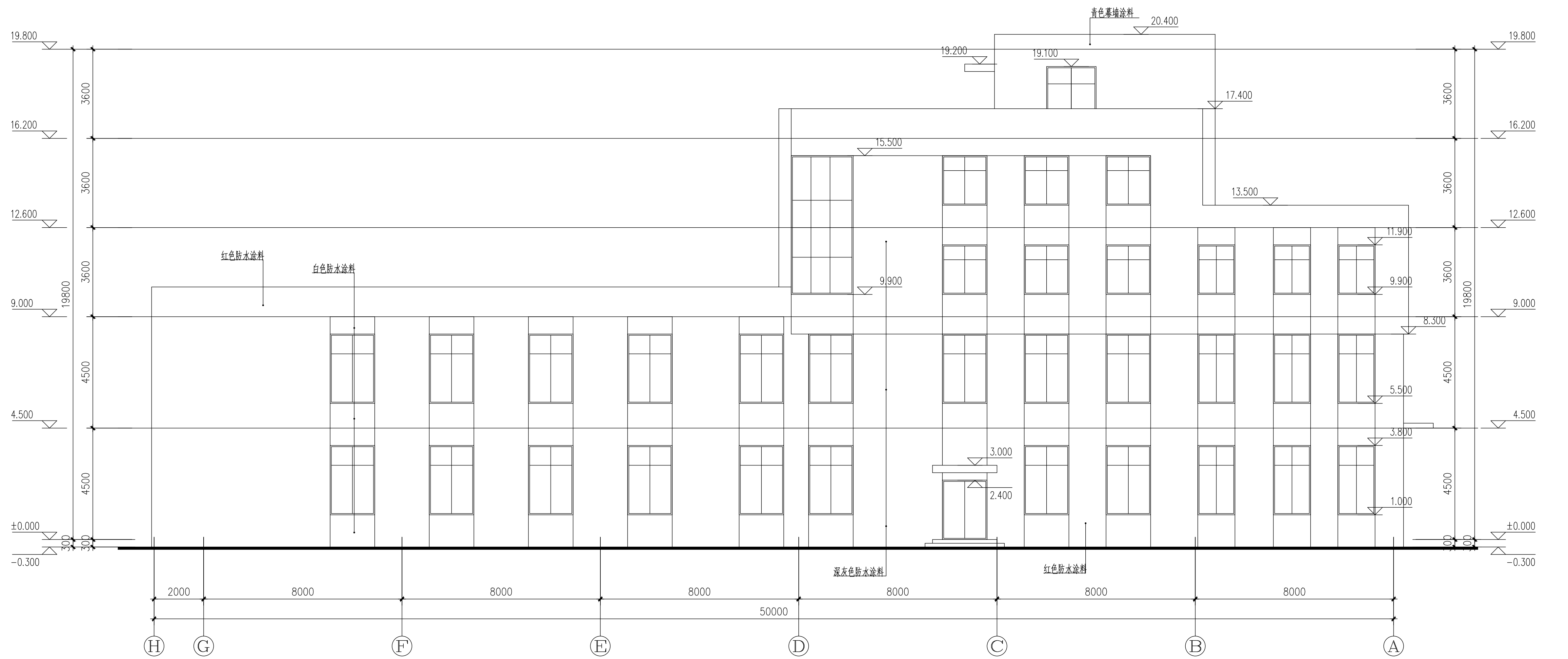
易安居西立面图125
