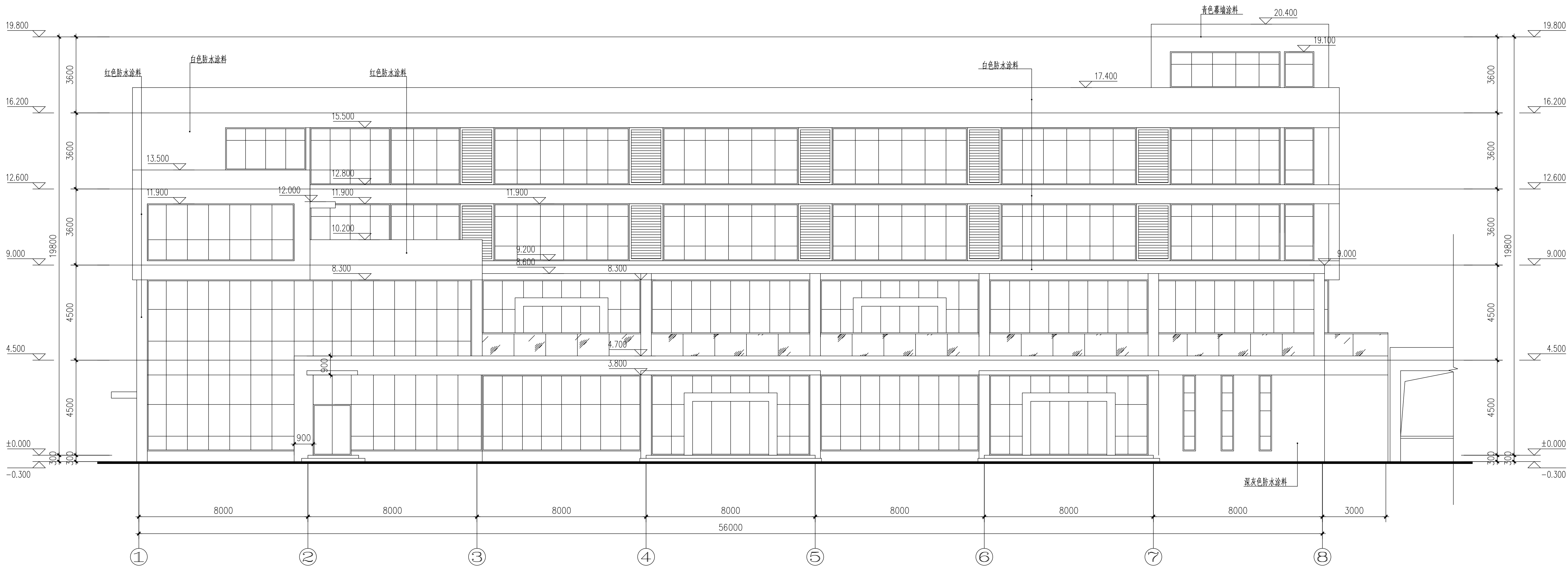
易安居南立面图25
