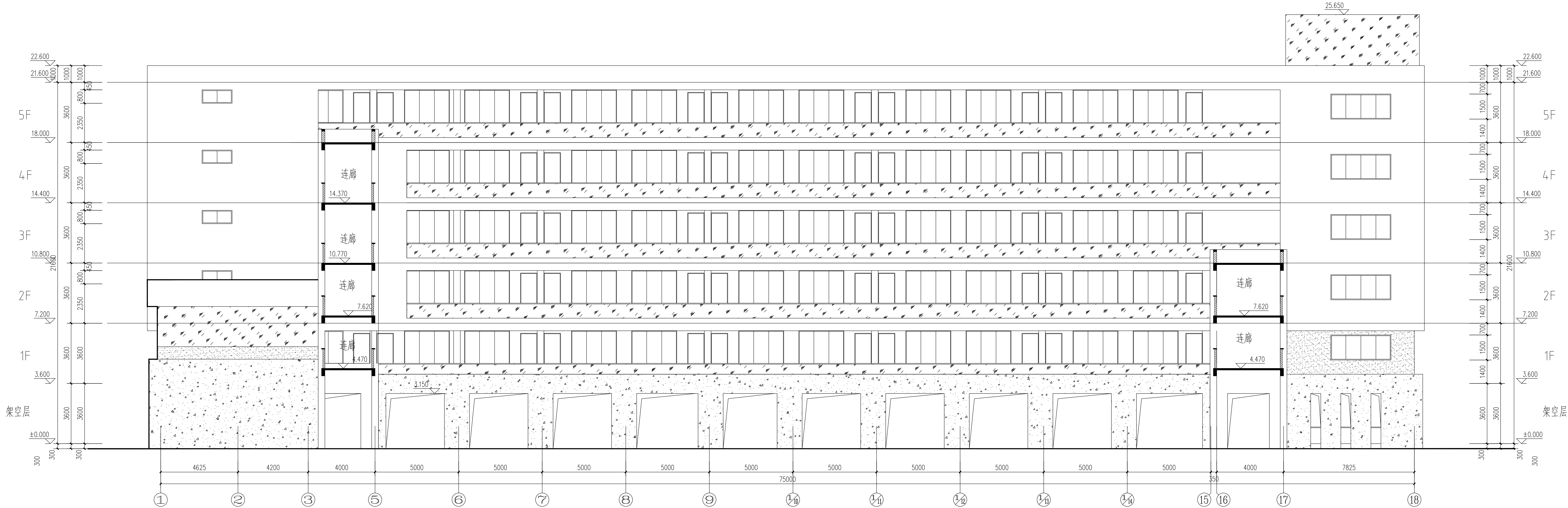
怀仁楼南立面图1:200
