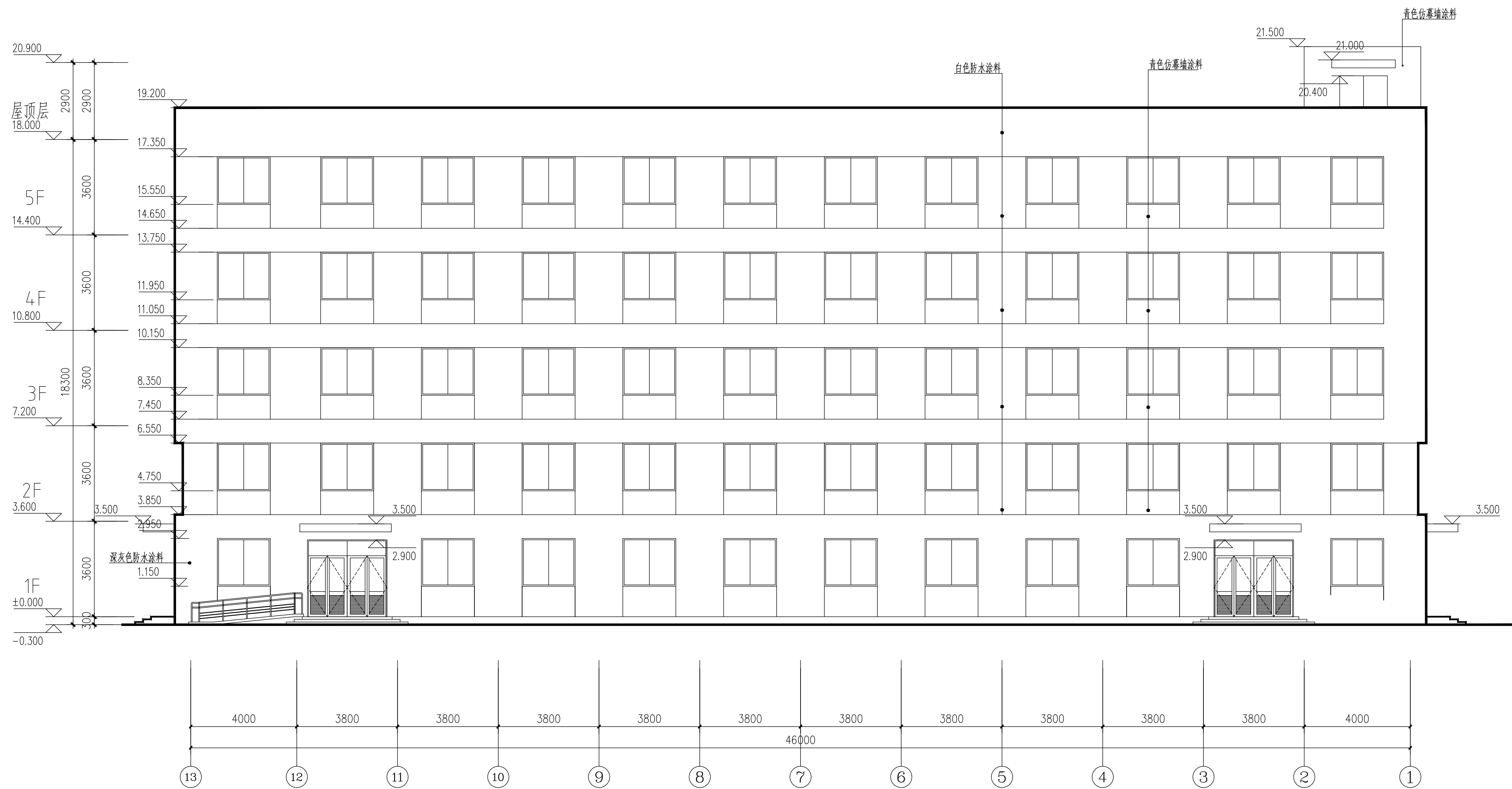
梦德轩宿舍楼北立面图:100 仅针对建筑外立面涂料改造
