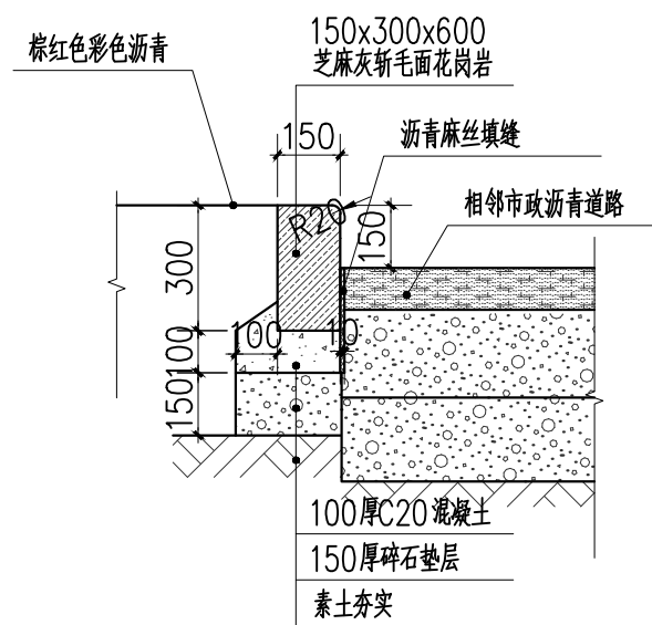
③人行道立缘石做法详图 1:25
