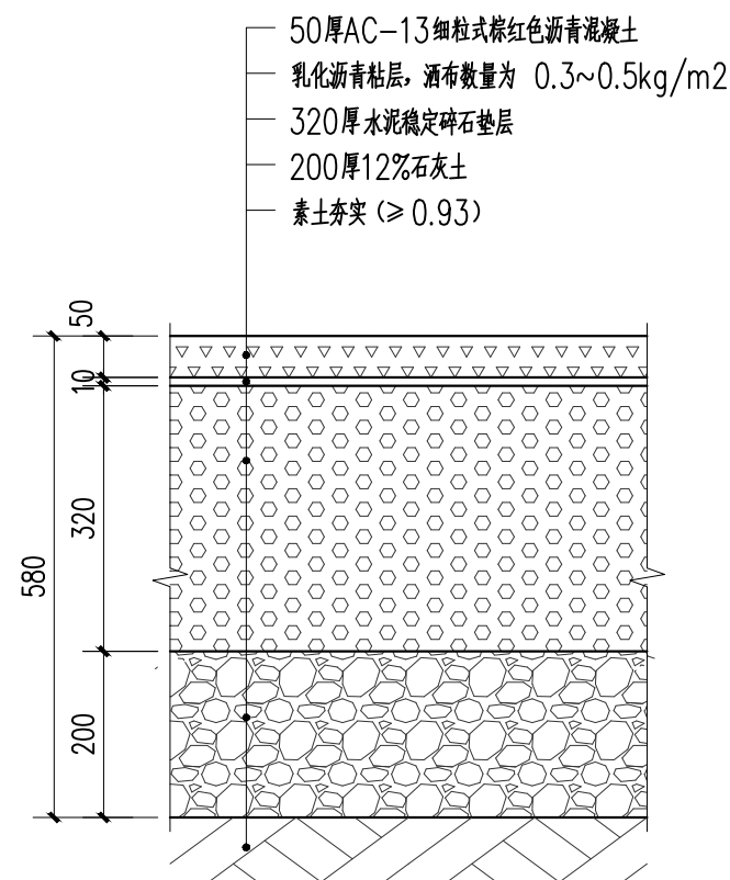
①人行道沥青路面做法详图 1:10
