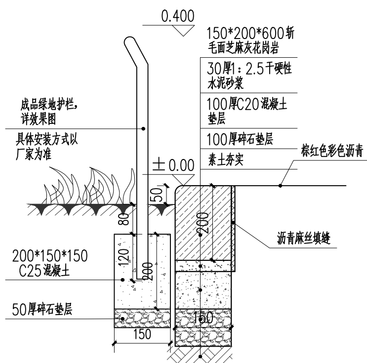
⑤绿地护栏及人行道平缘石详图 1:10
