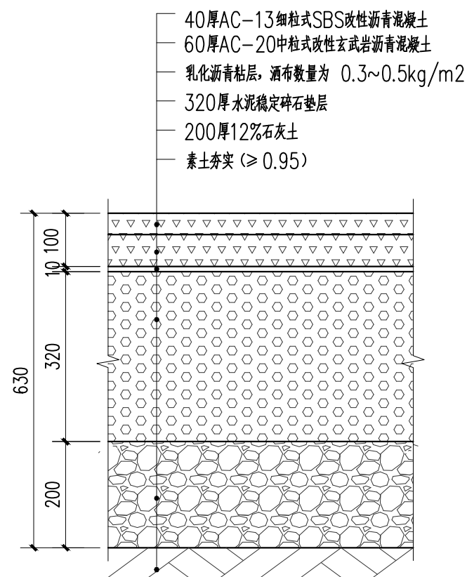
②停车场沥青路面做法详图 1:10
