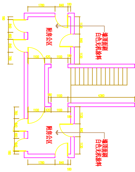
附房至一层 (二三单元)
