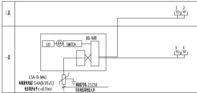
综合布线系统图
