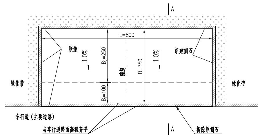
类型 (C) 停车棚平面 (1/2) 1:100 适用于新建停车棚临近小区内主要交通道路
