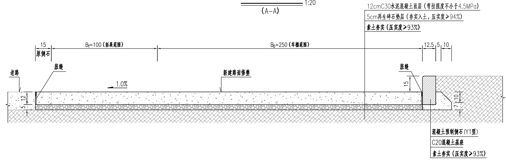
(每个)类型 (C) 停车棚材料数量表 B 1 =100cm
