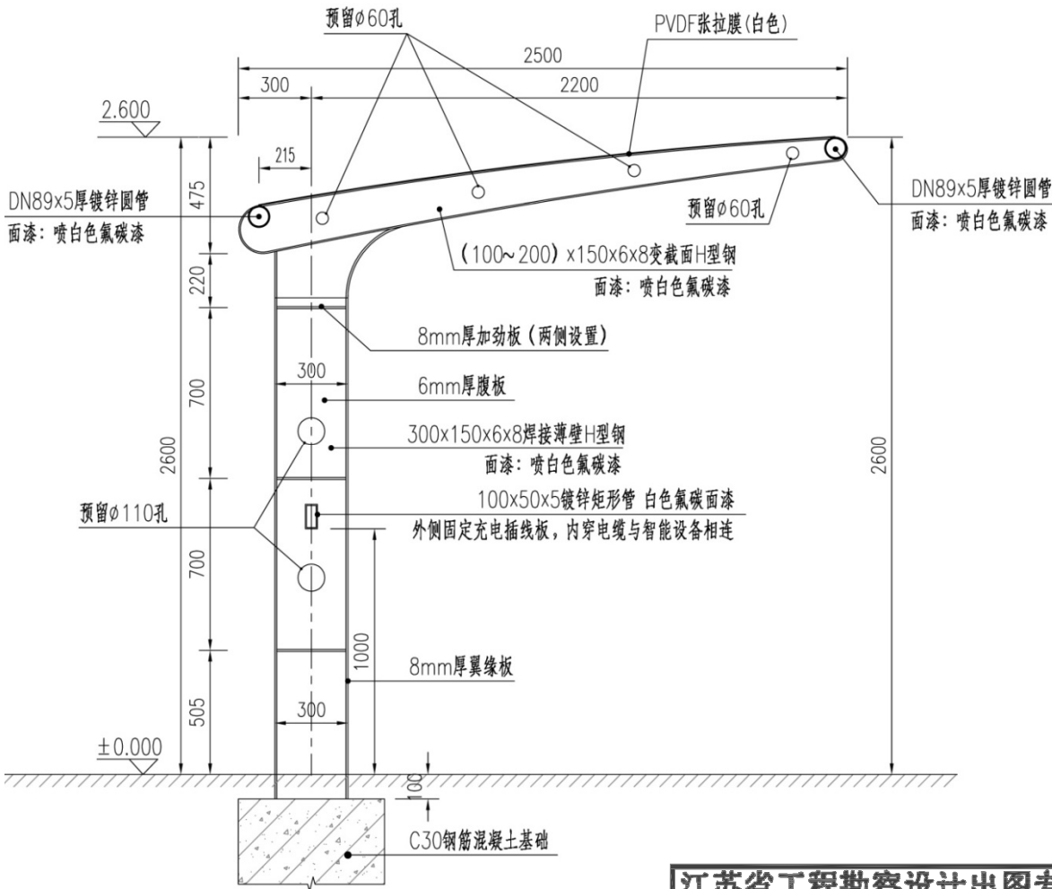
图 5-1 车棚剖面图（
