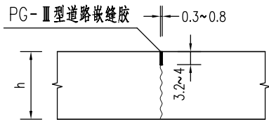
胀缝构造图
