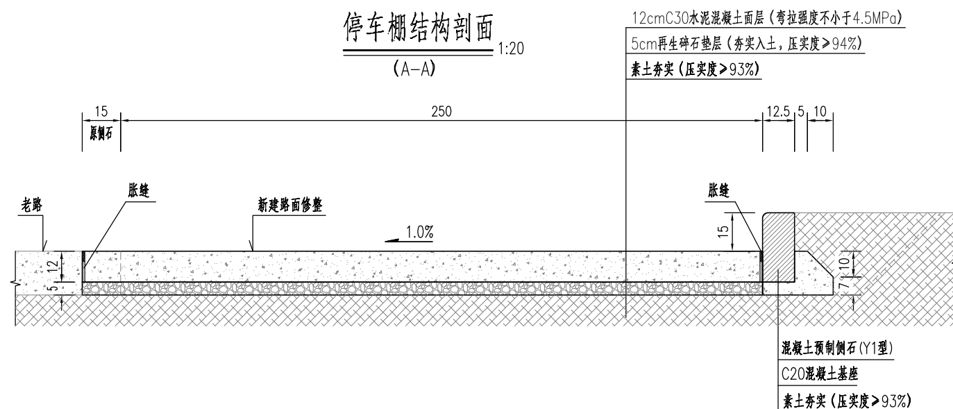
分类 材料名称 规格 单位 数量 新建 混凝土 场地 C30水泥混凝土面层 h=12cm m 2 31.80 再生碎石垫层（夯实入土） h=5cm m 2 31.80 侧石 75x27x12.5 m 17.00 侧石C20基础 m 3 0.46 胀缝 m 29.00 缩缝 m 5.00 拆除 挖方 拆除侧石 m 12.00 绿化土方 m 3 13.08
