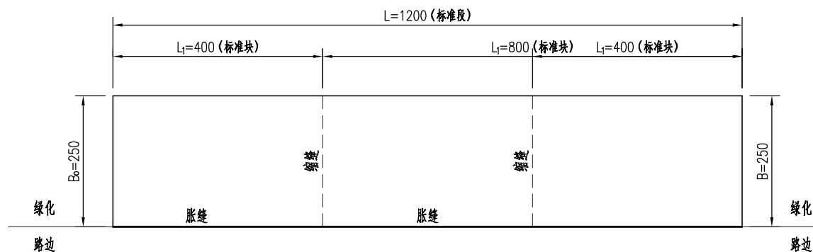
类型(D) 板块划分平面图
