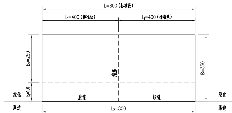
类型(C) 板块划分平面图
