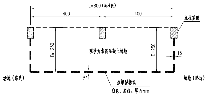
类型(D) 板块划分平面图
