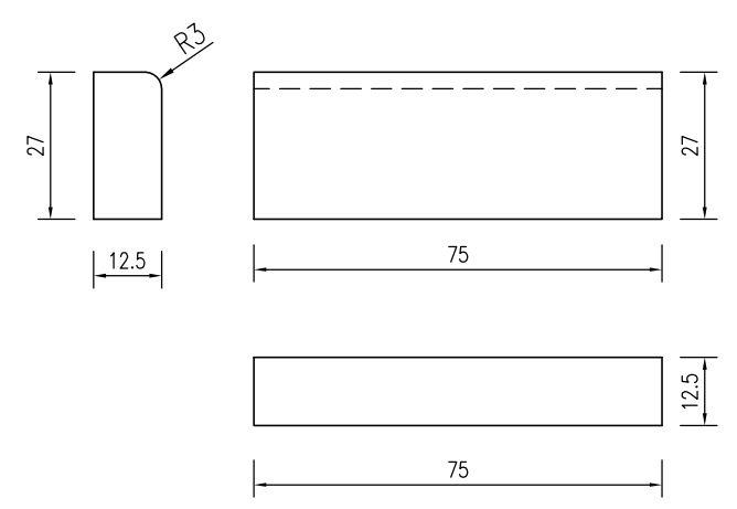
Y1侧石构造 1:15
