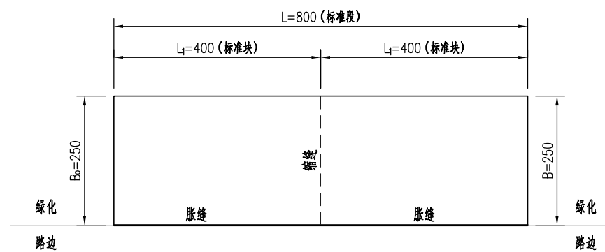
类型(A) 板块划分平面图
