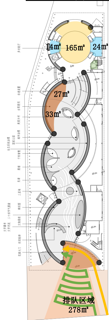
首层平面图 1F
