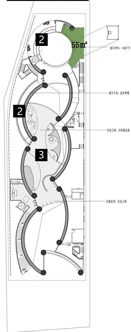
二层平面图 2F
