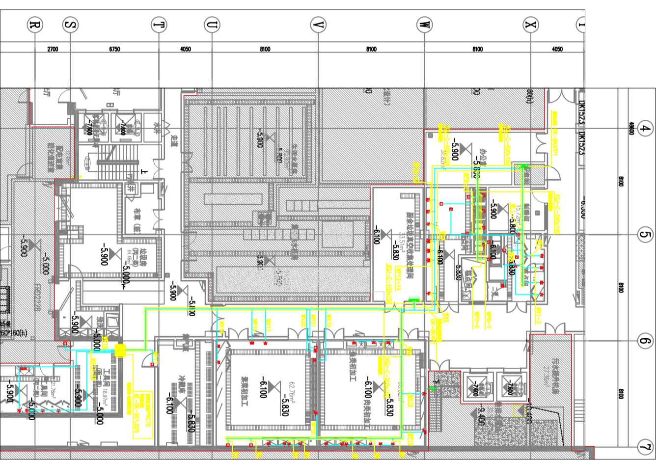
地下二层电位配电平面图 1:100
