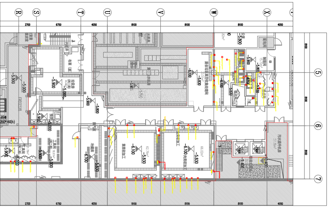
地下二层电位平面图 1:100
