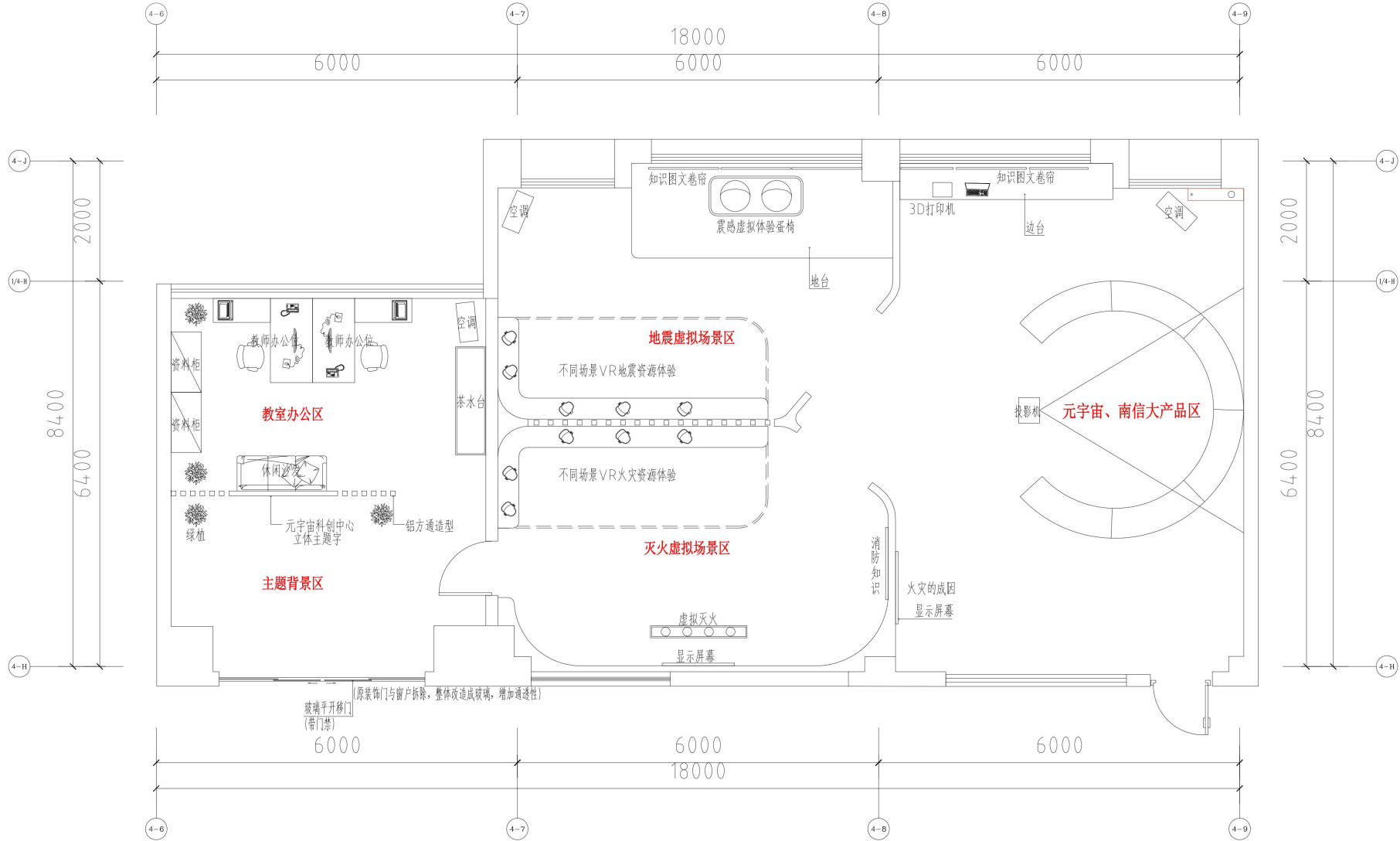
元宇宙科创中心平面布置方案
