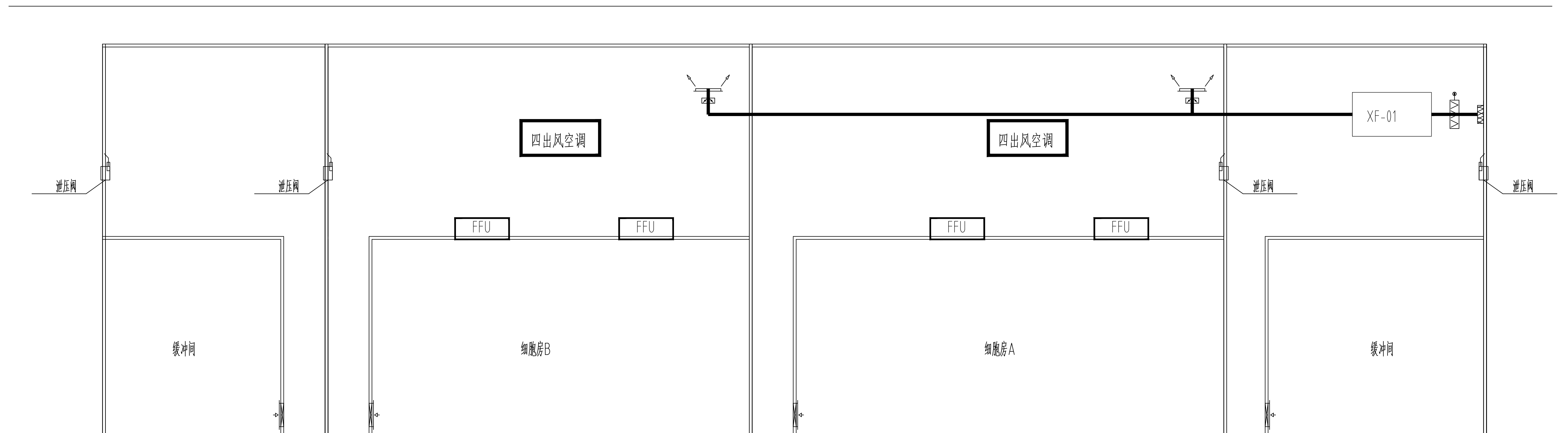
细胞房风系统流程图
