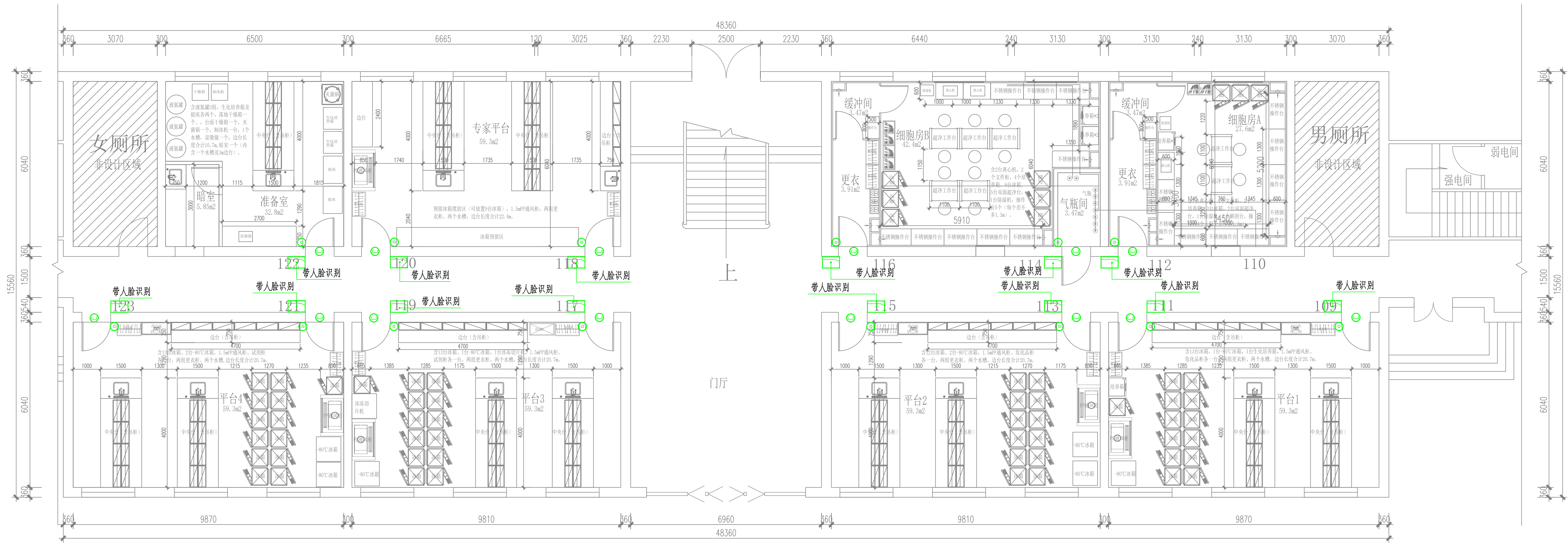
6号楼门禁平面布置图
