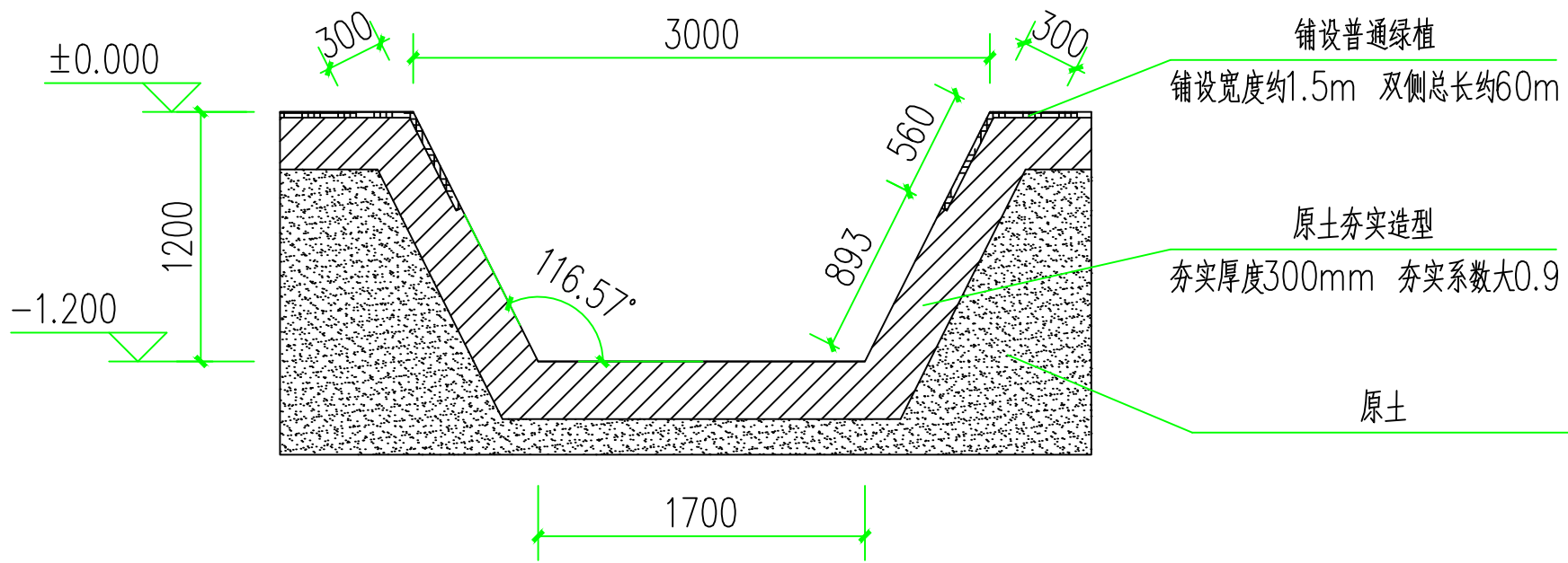
河道一 4-4剖面图
