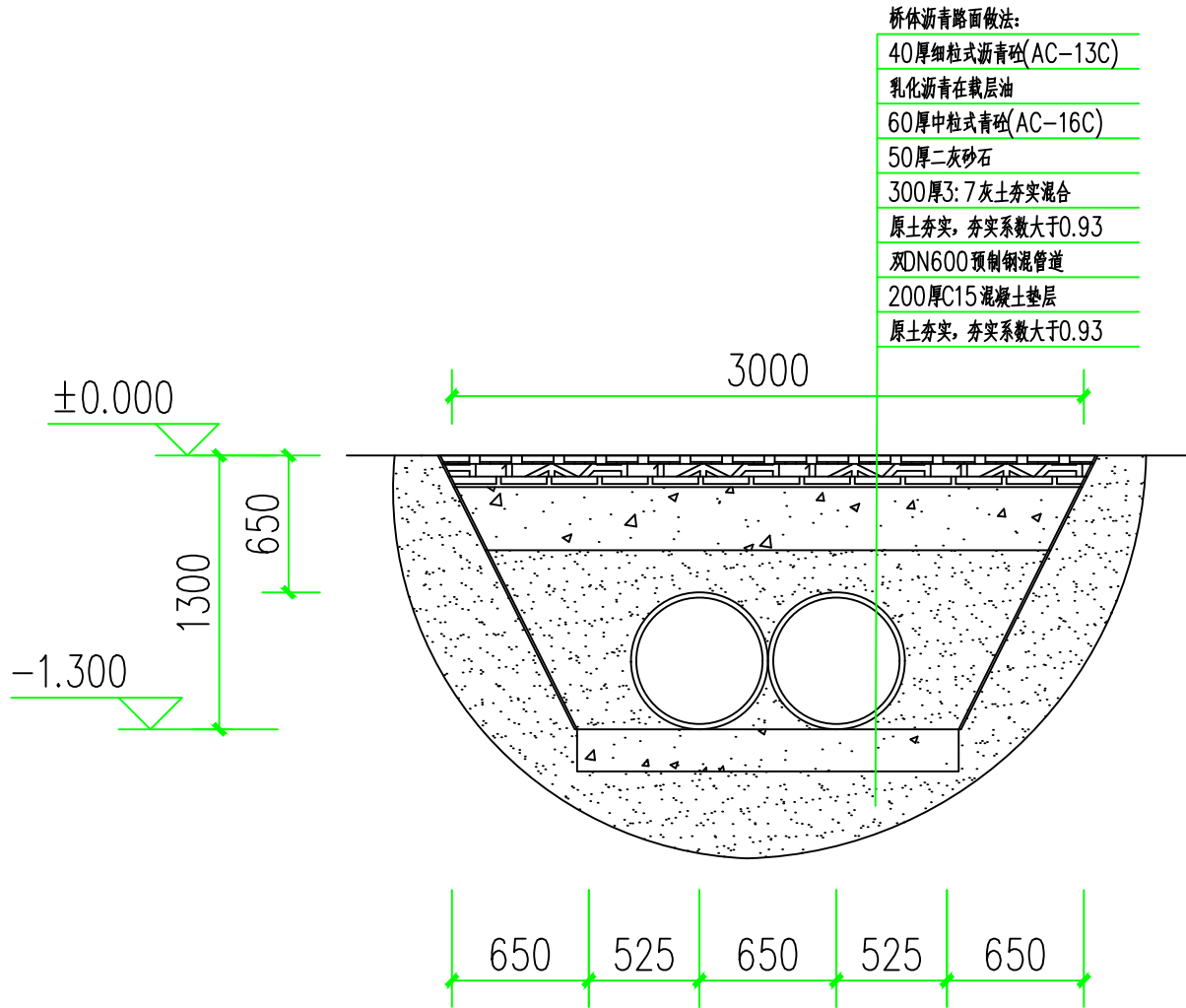
河道一 3-3剖面图
