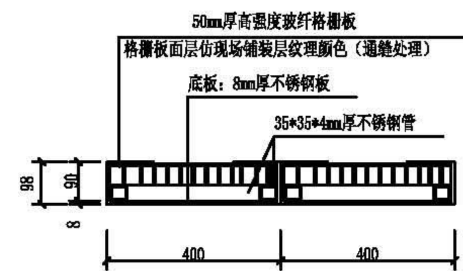
井盖侧面图
