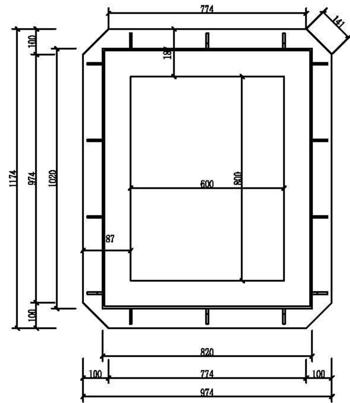
井框平面图
