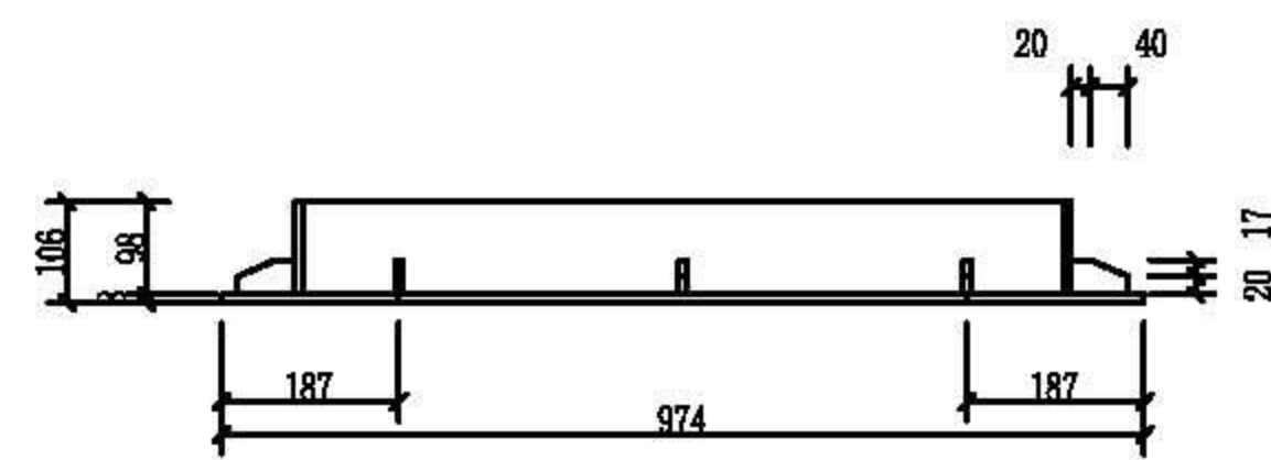
井框侧面图
