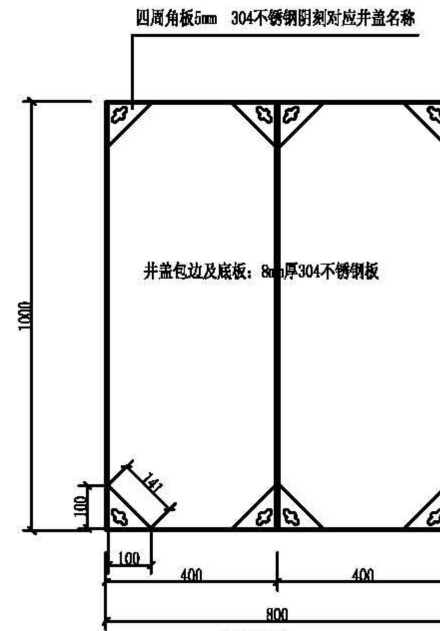
井盖平面图
