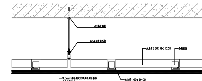
空调拆改吊顶修补通用节点2
