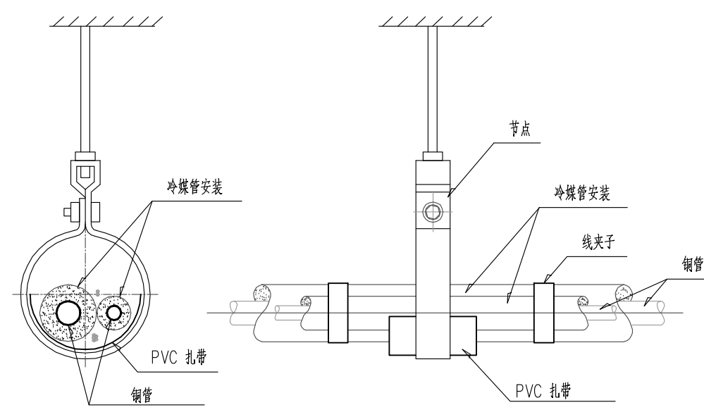
铜管吊装大样图
