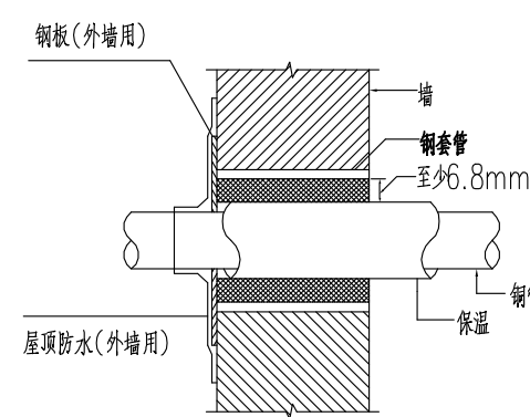
铜管过墙安装大样图
