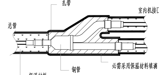
分歧管安装大样图
