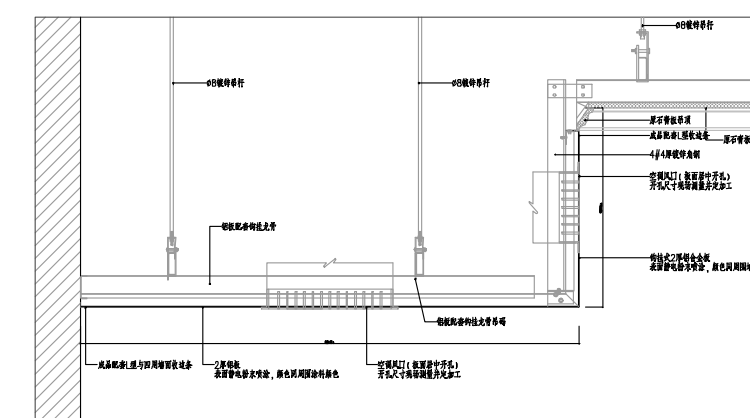
空调拆改吊顶修补通用节点
