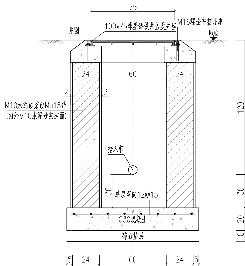
弱电手工井侧面图 1:20
