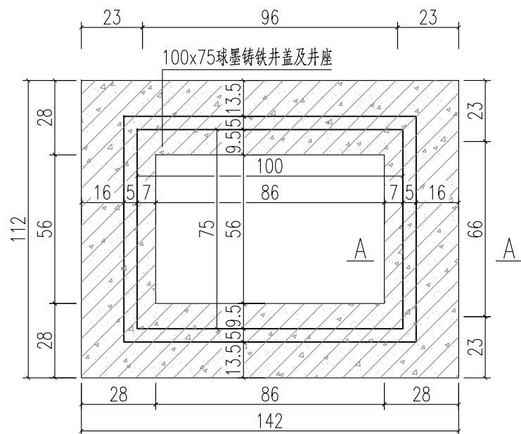
井圈平面图 1:20
