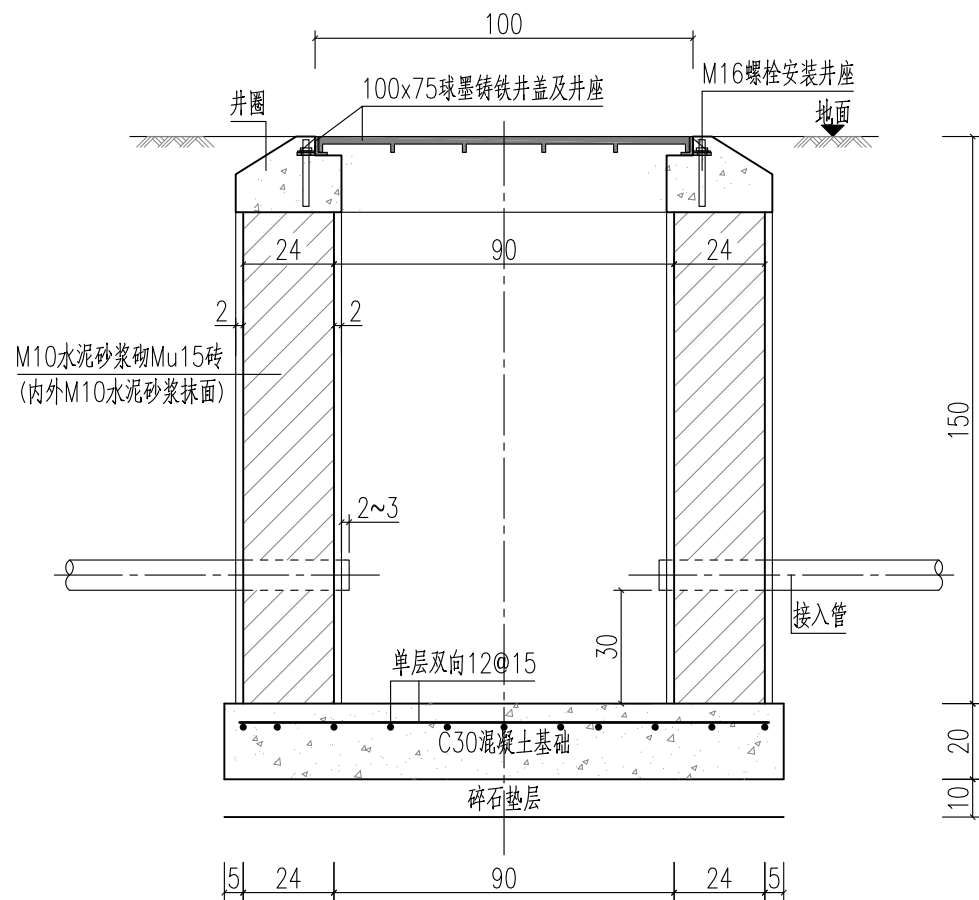
弱电手工井立面图 1:20
