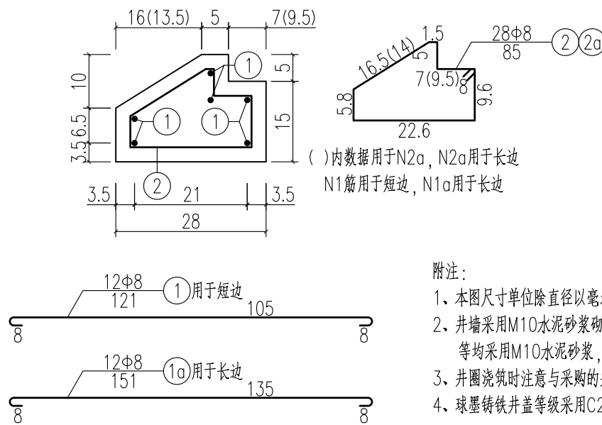
A-A 1:10
