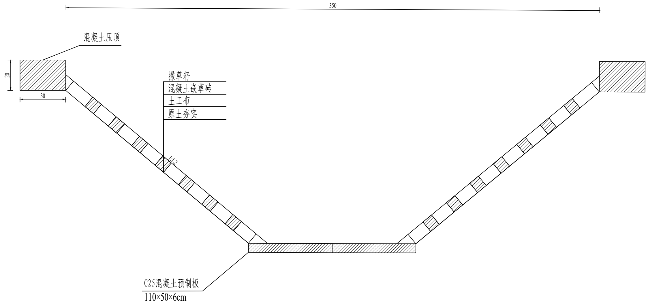
生态沟横断面设计图
