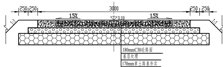
碎石道路标准断面图
