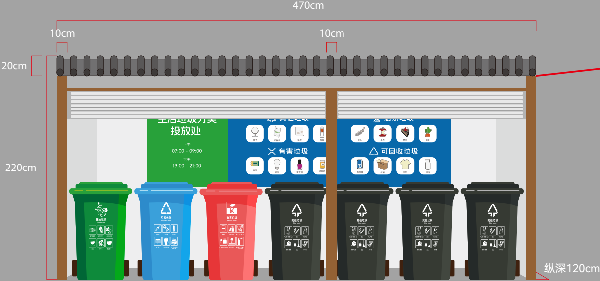
7个垃圾桶
