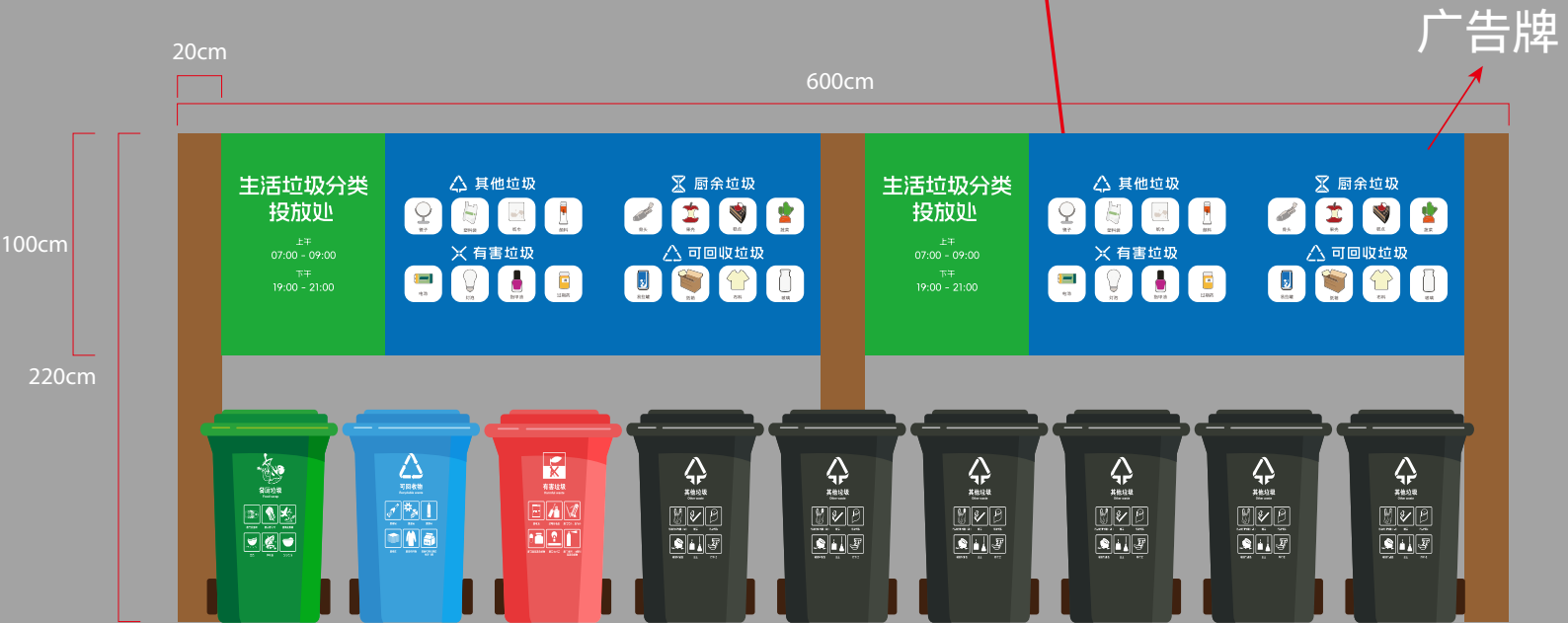
9个垃圾桶
