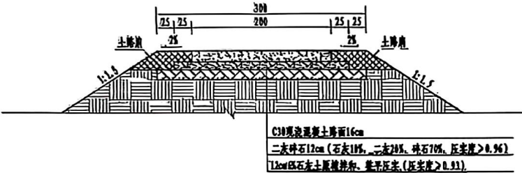
2.0m宽混凝土道路典型断面图
