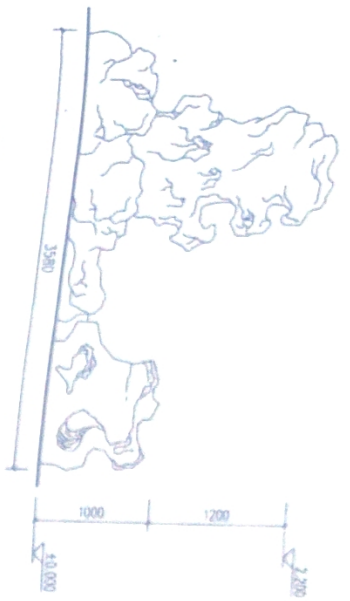
1 成品太湖石一立面图 1:30
