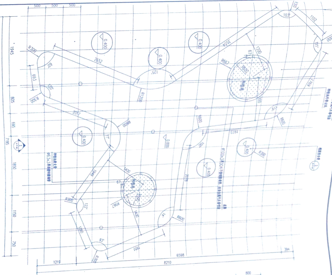
1 2-1 树池桌子坐凳三平面图 1:30
