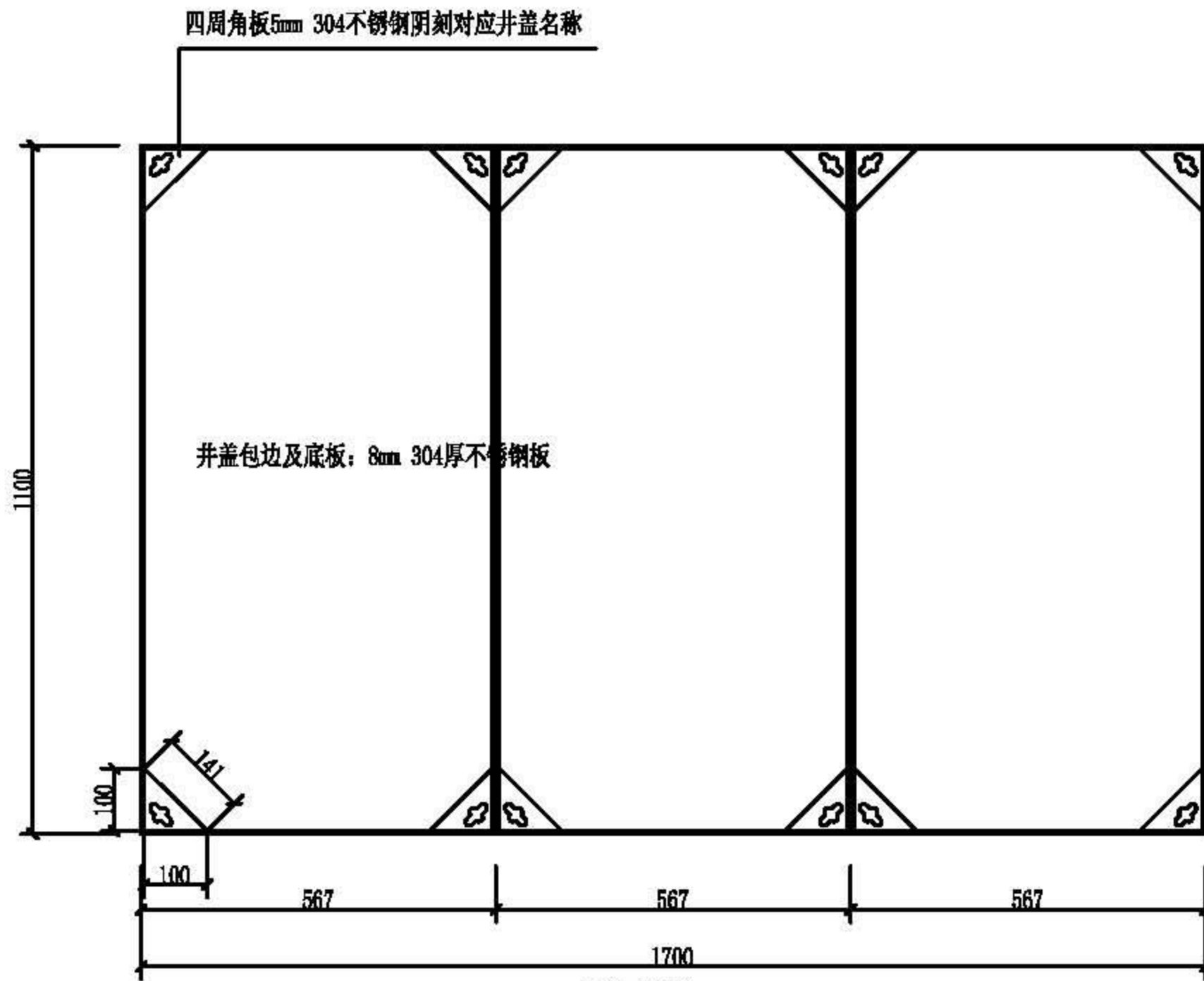
井盖平面图
