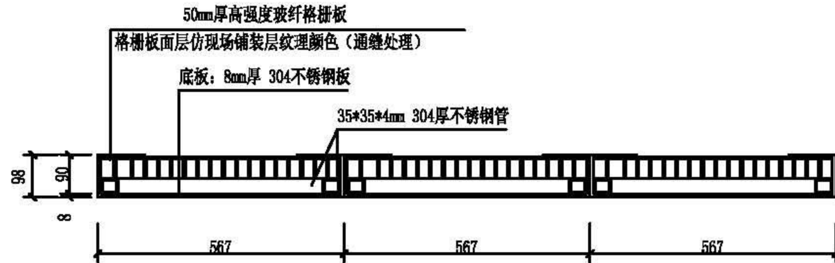
井盖侧面图
