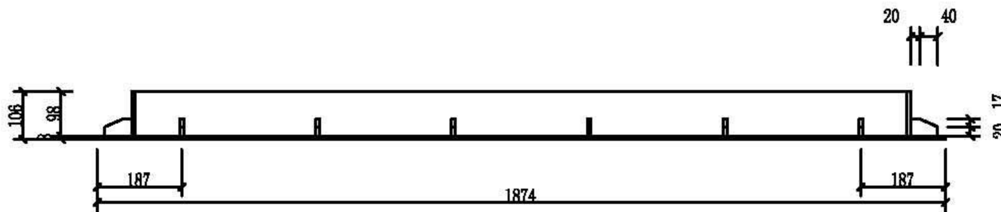
井框侧面图
