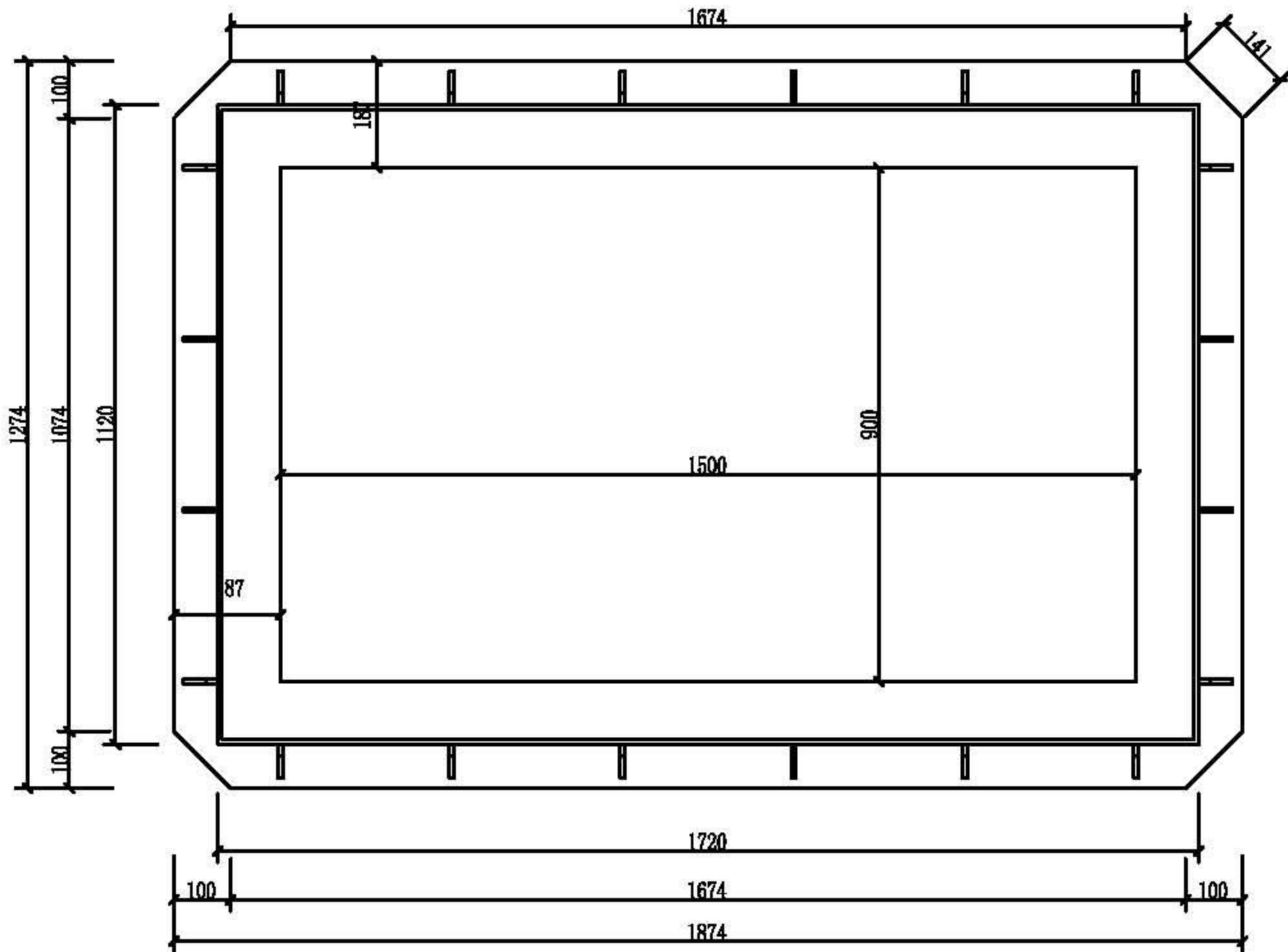
井框平面图
