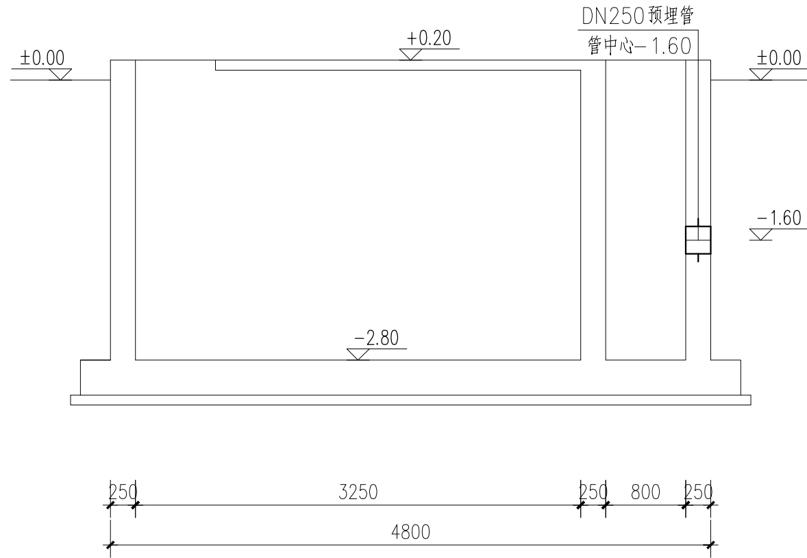
格栅井/调节池B-B剖面图
