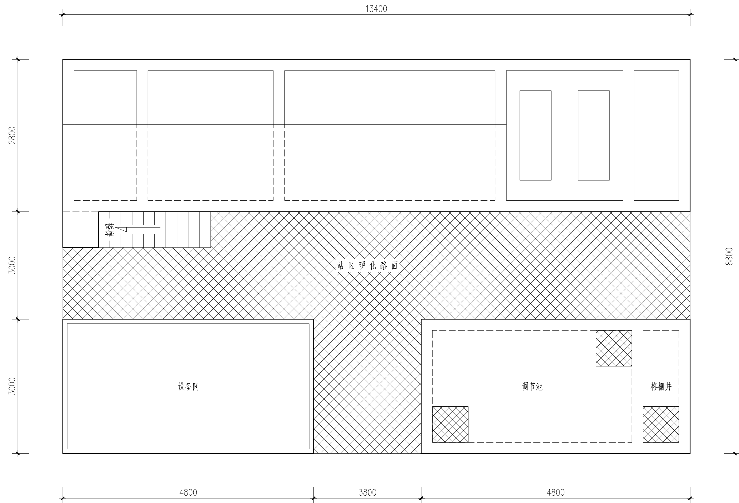
100吨/日污水处理站平面布置图
