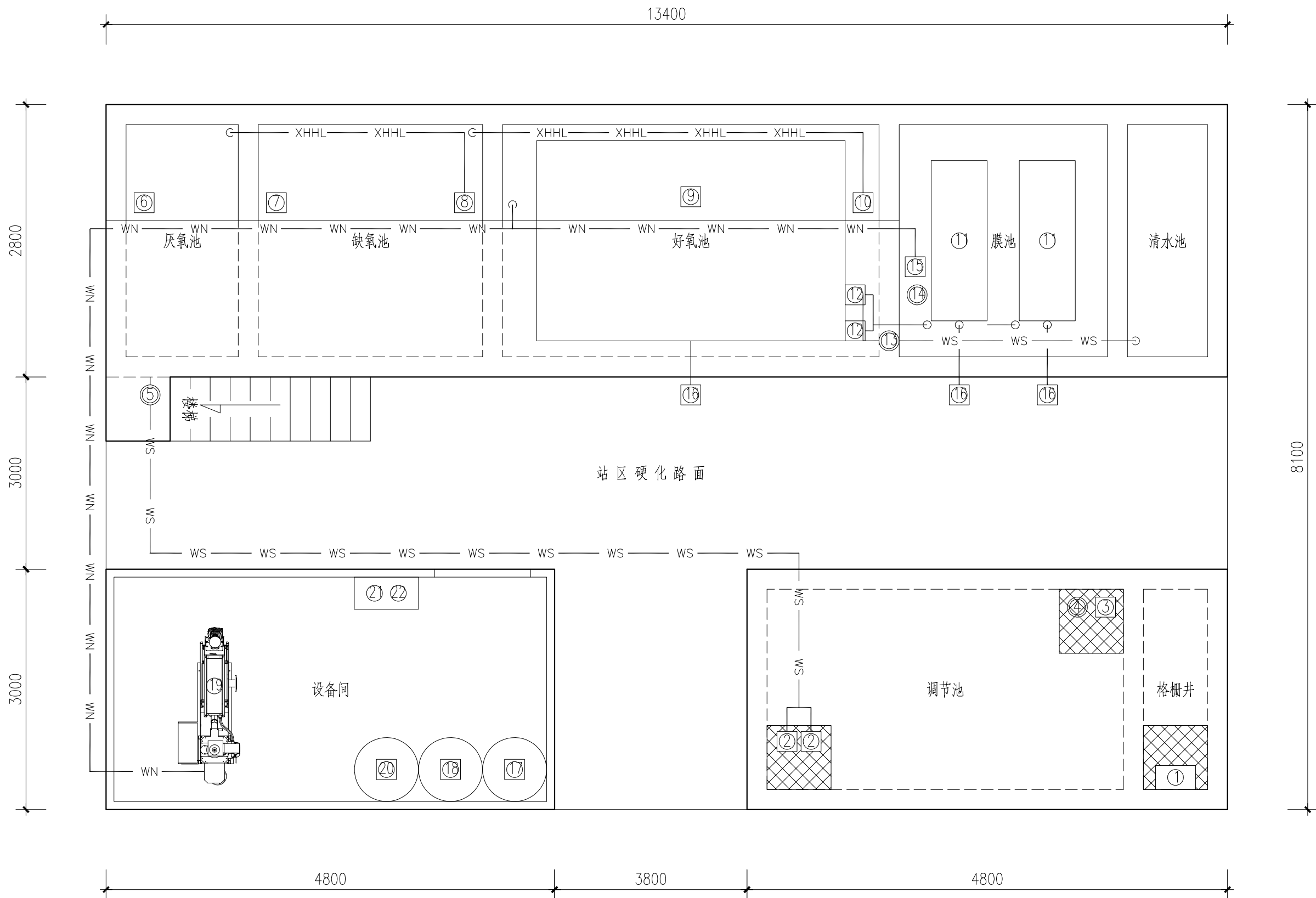
100吨/日污水处理站设备布置图
