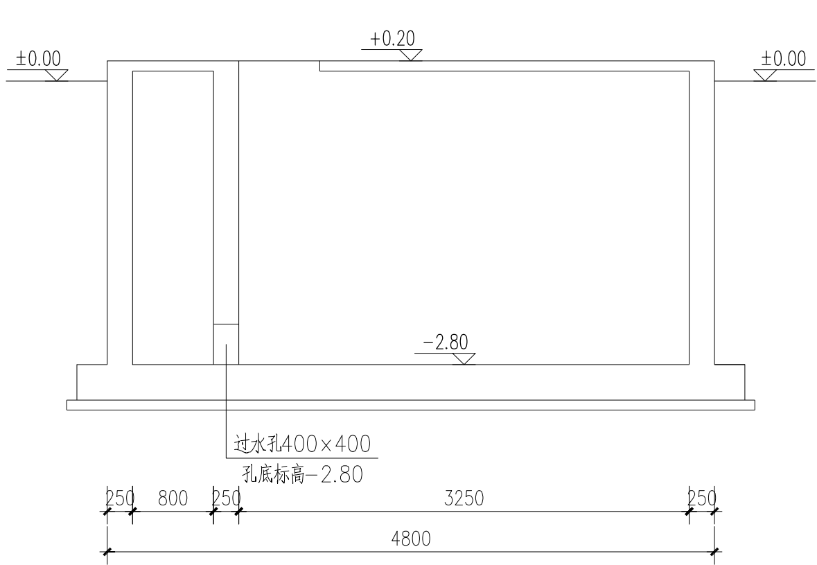
格栅井/调节池A-A剖面图
