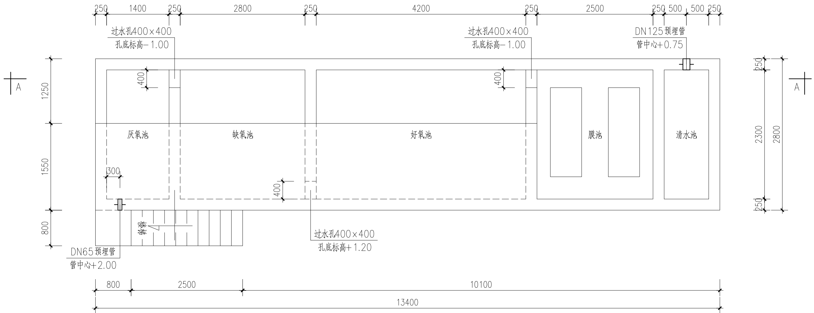
一体化生化池平面图
