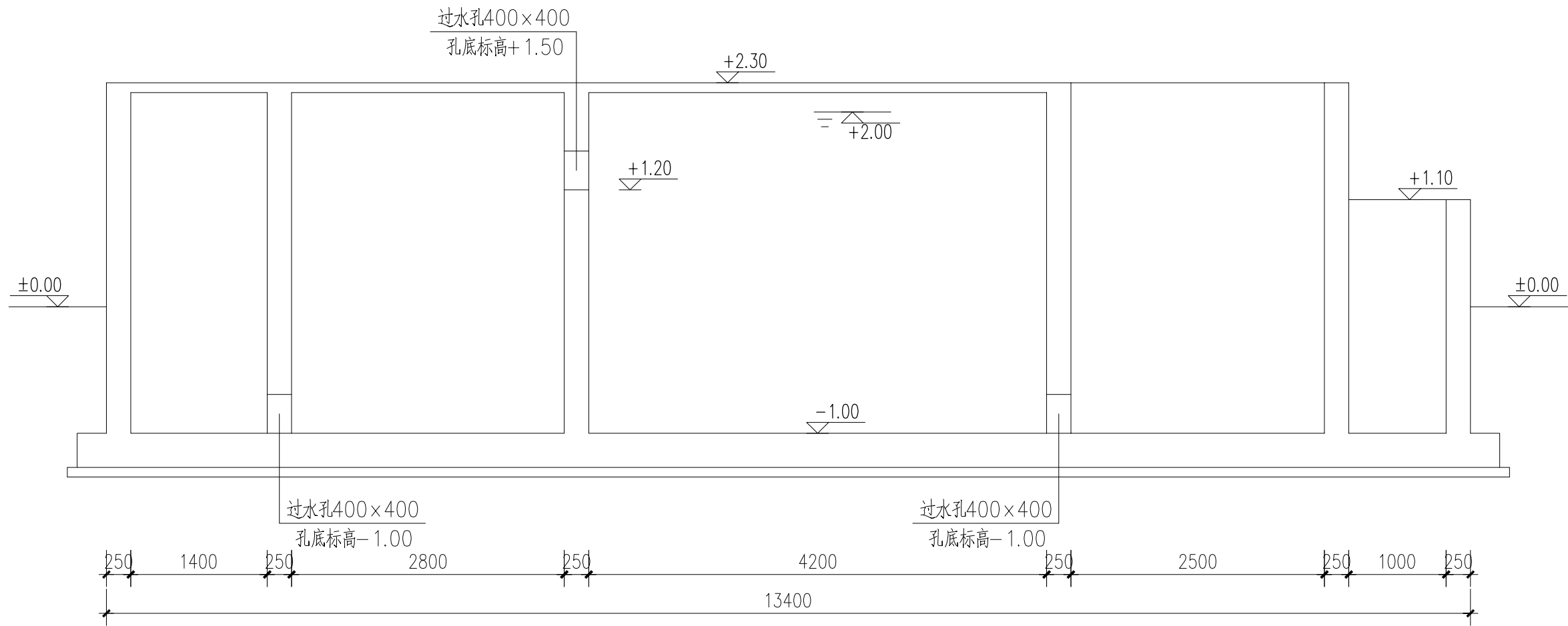
一体化生化池A—A剖面图
