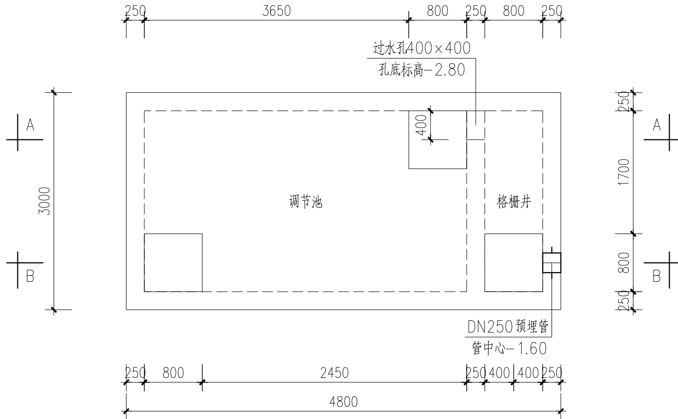
格栅井/调节池平面图
