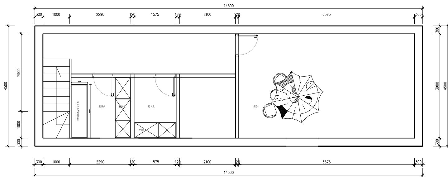
二层平面布置图
