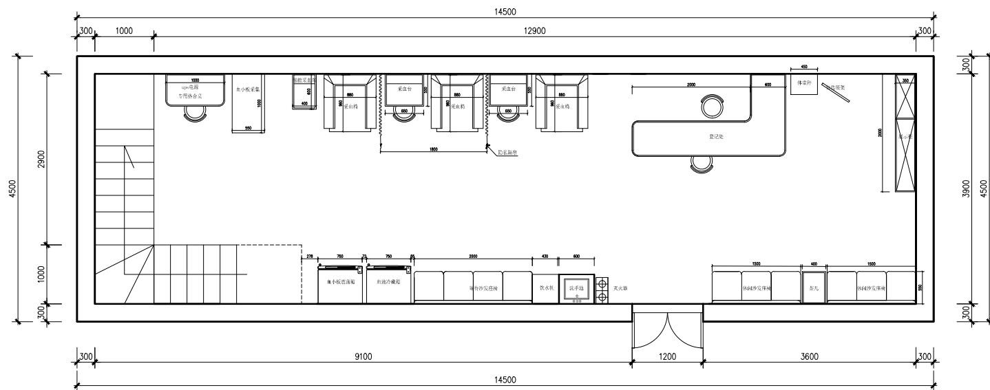
一层平面布置图
