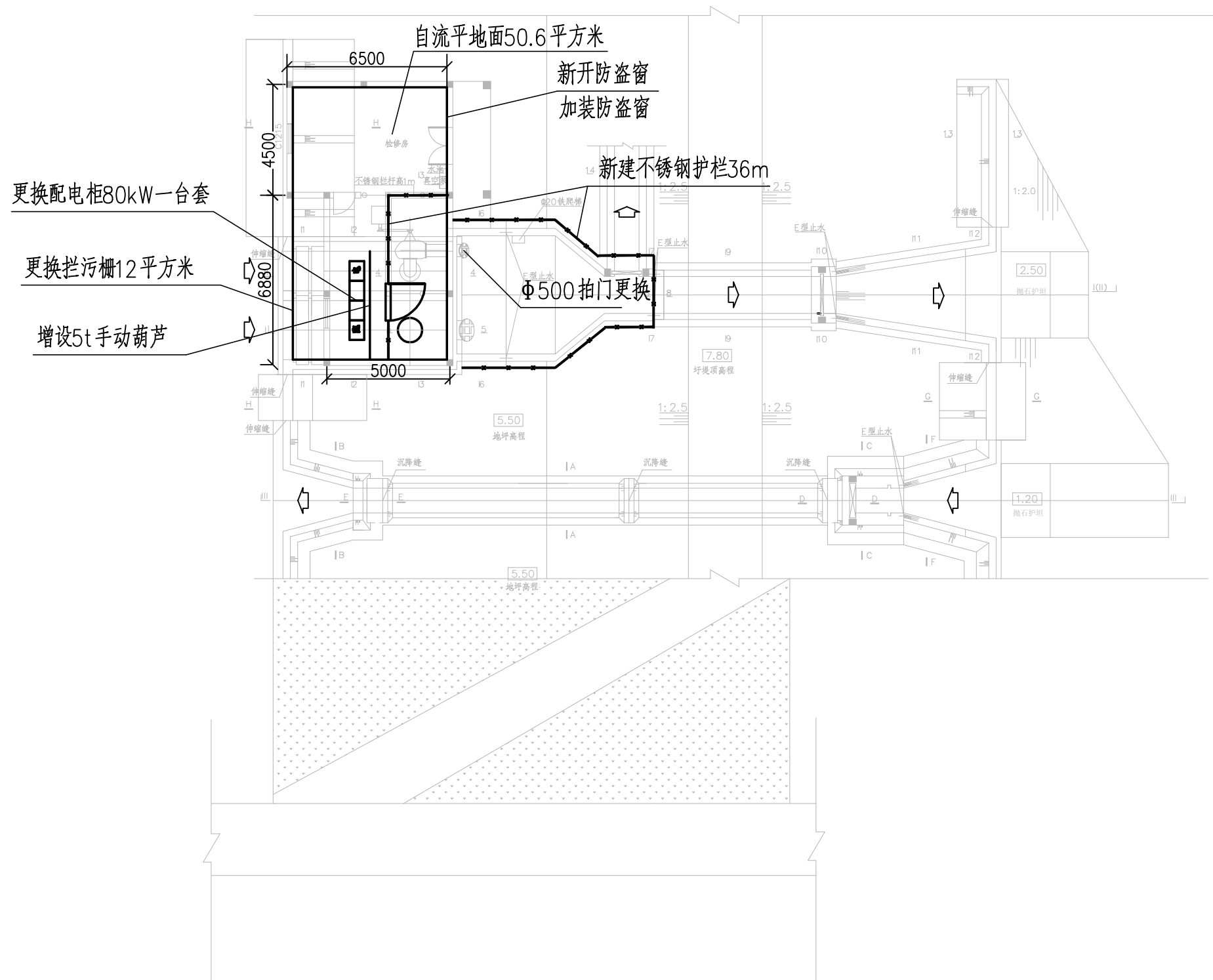
平面布置图—扁担河排灌站 1:200
