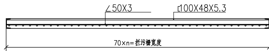
d-d剖面结构图 1:50
