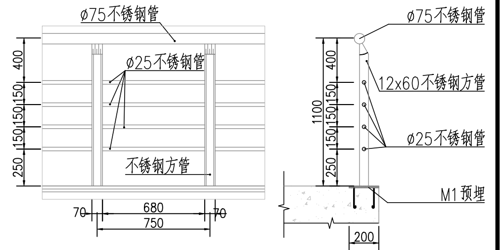
不锈钢栏杆结构图 1:25
