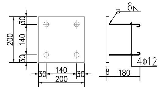
M1 1:25
