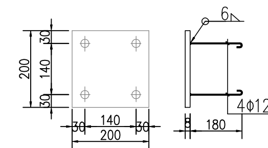
M1 1:25
