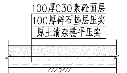
素砼场地 1:50
