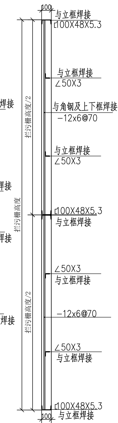
c-c 剖面结构图 1:50
