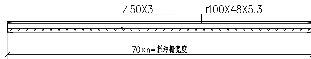
d-d 剖面结构图 1:50
