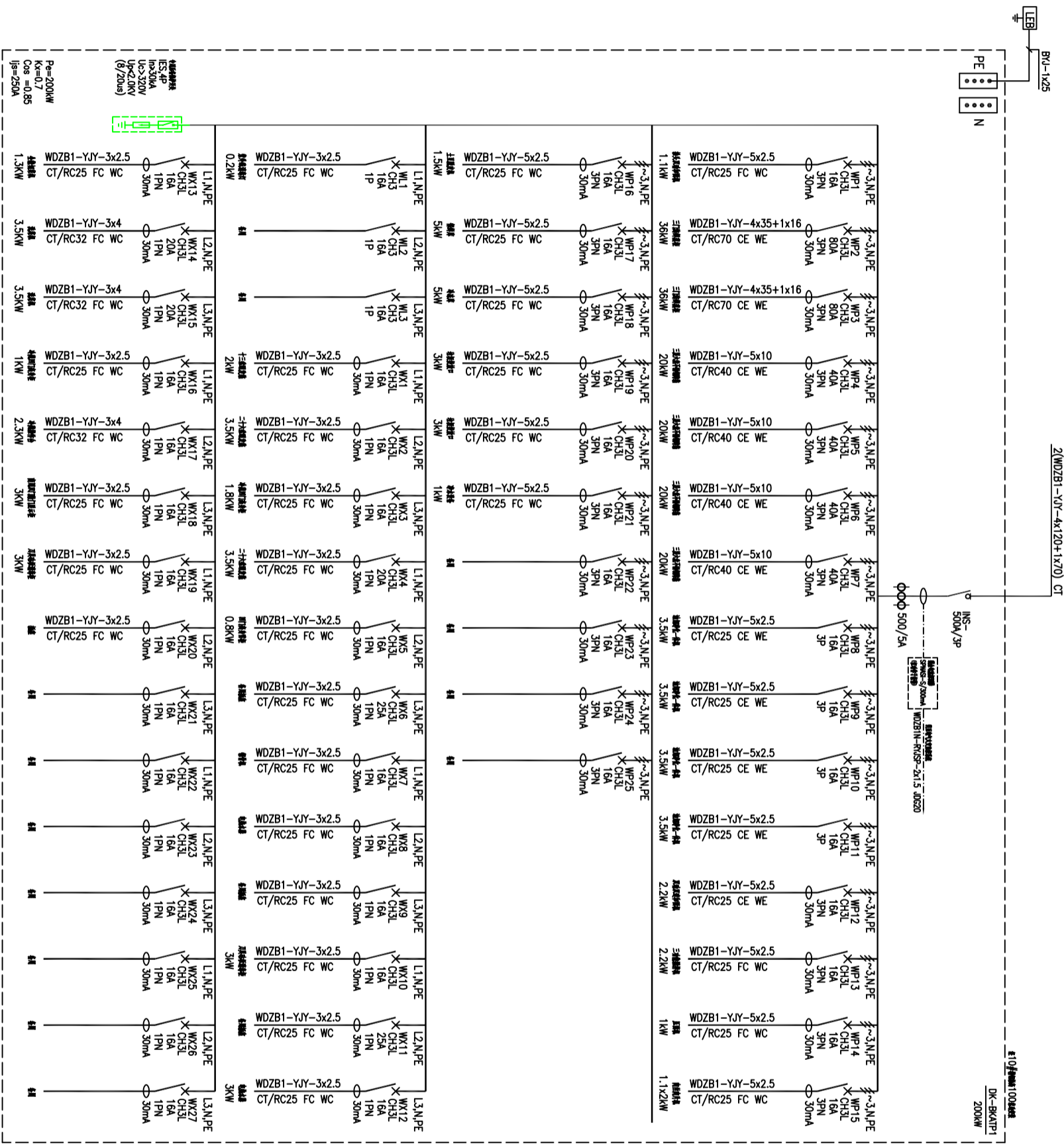
配电箱系统图 DK-BKATP1 系统图
