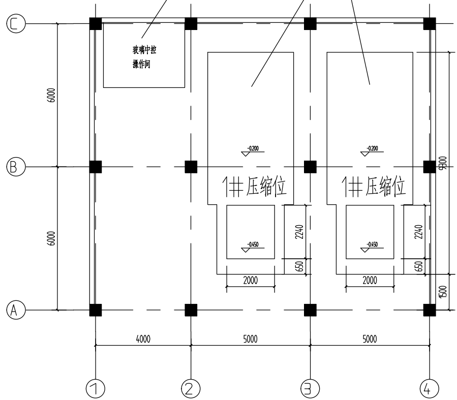
整改建筑平面图
