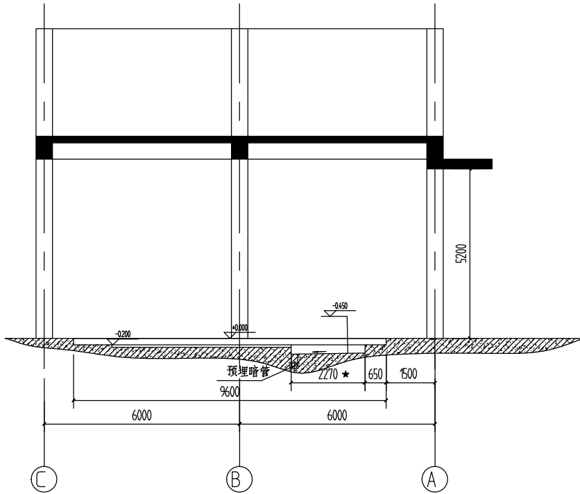
整改建筑立面图
